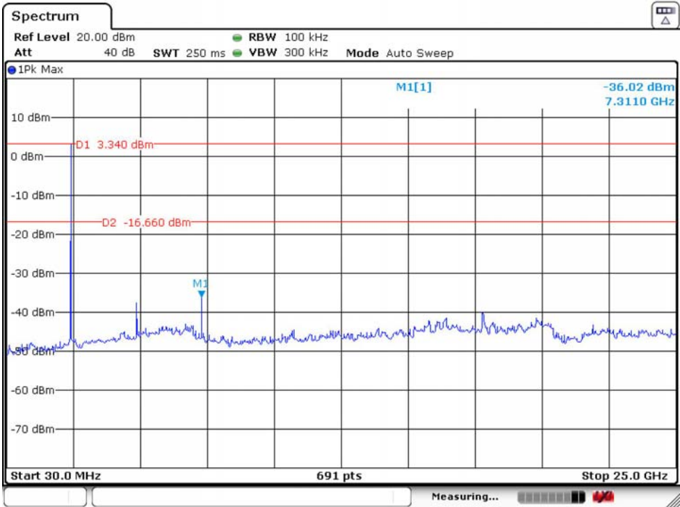
GFSK 2441 MHz
