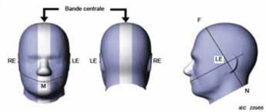
Illustration du fantôme donnant les points de référence des oreilles, RE et LE, le point de référence de la bouche, M, la ligne de référence M-F et la bande centrale
