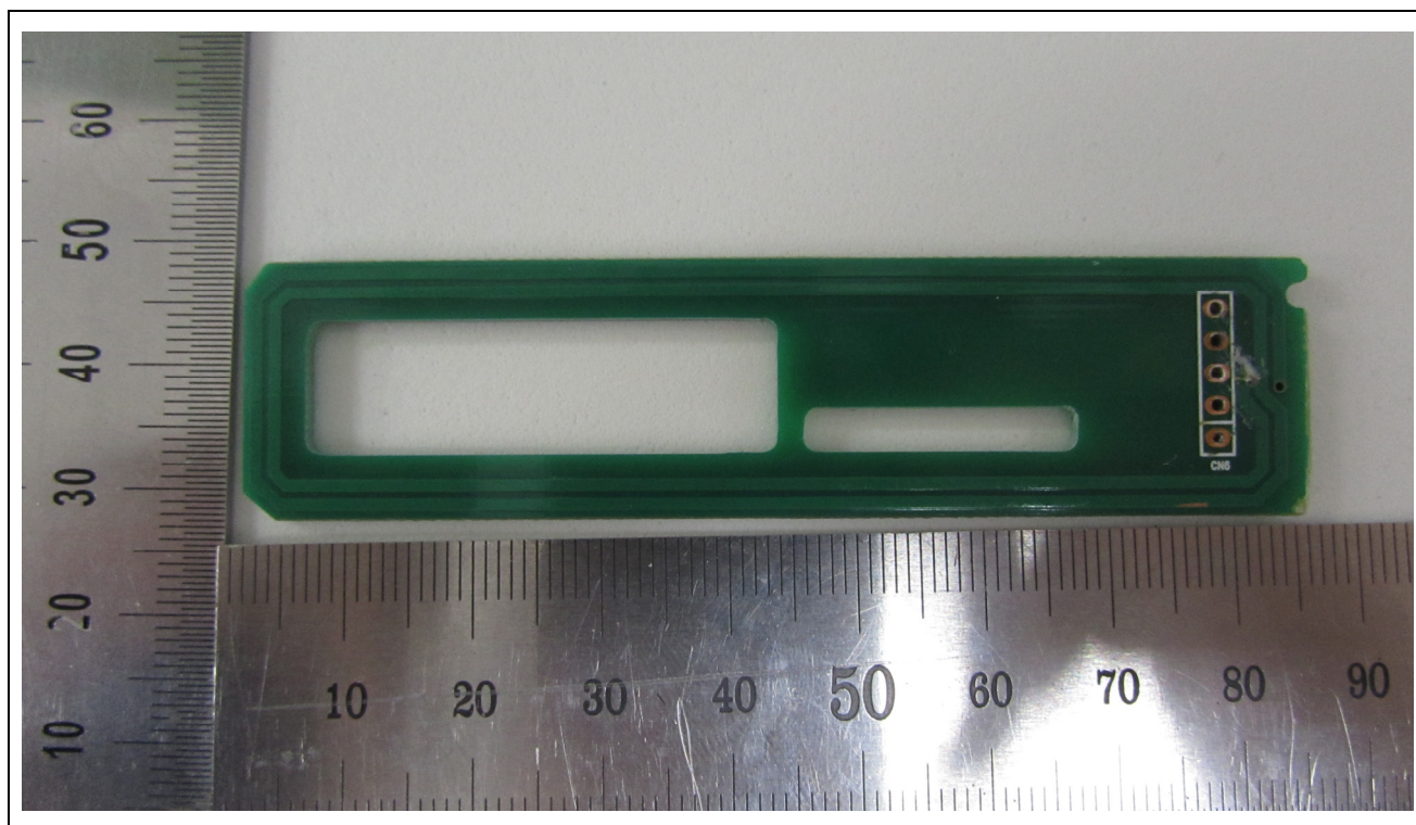
<Antenna>
