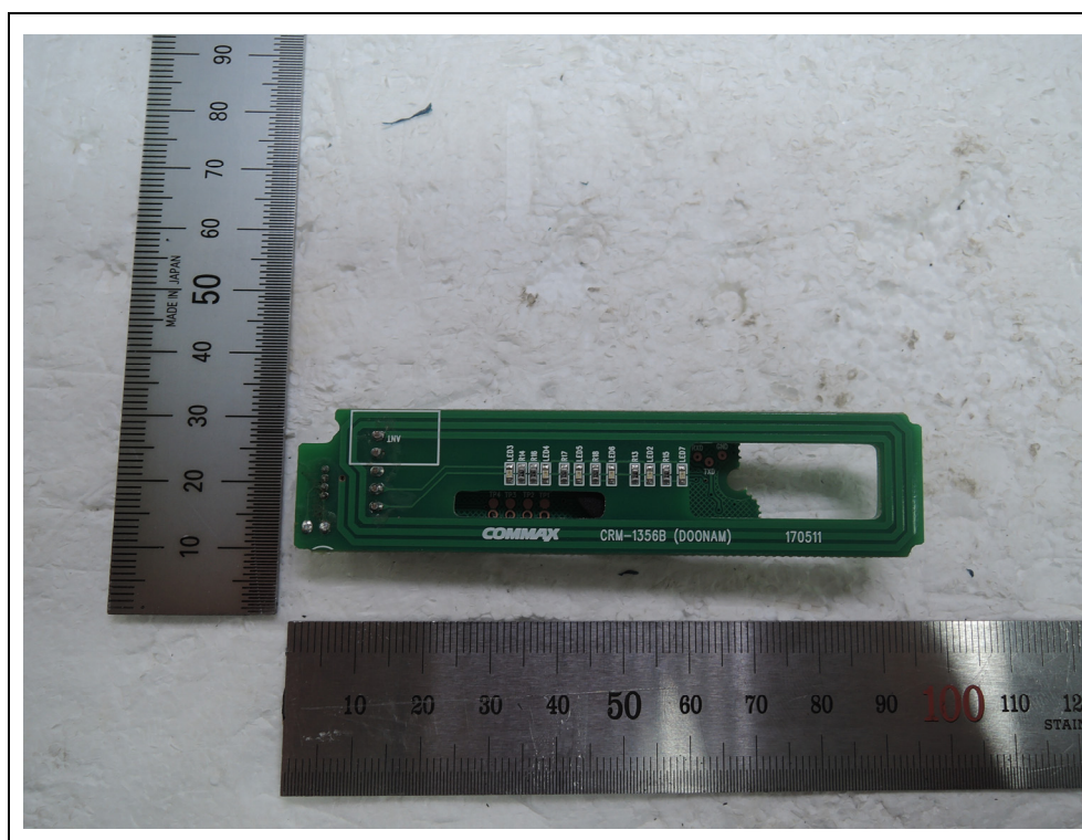
<Antenna>
