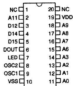
HT6187 - 20 SOP
