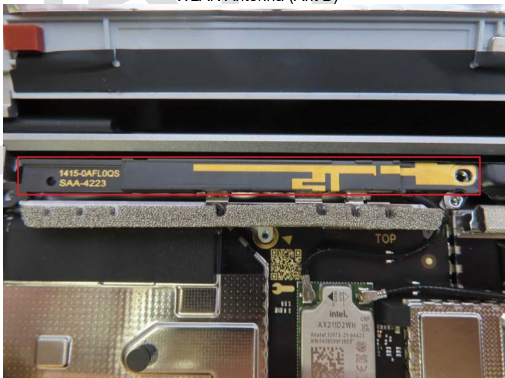
WLAN Antenna (Ant B)
