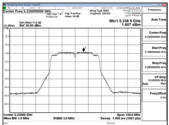
802.11n_40MHz_5230MHz-5230
