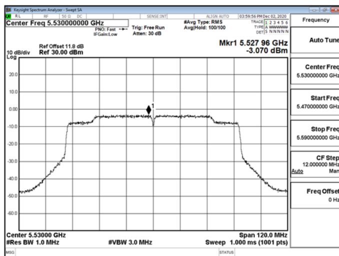
802.11ac_80MHz_5530MHz-5530
