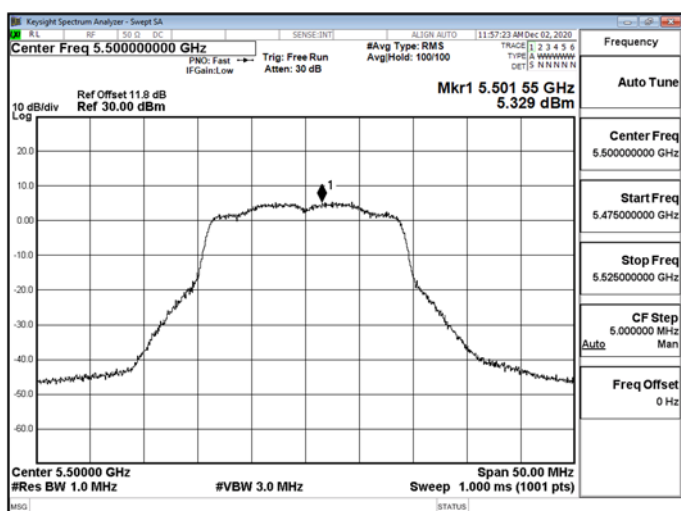
802.11n_20MHz_5500MHz-5500
