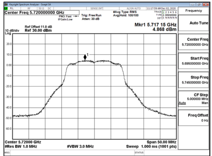
802.11a_20MHz_5720MHz_UNII 3
