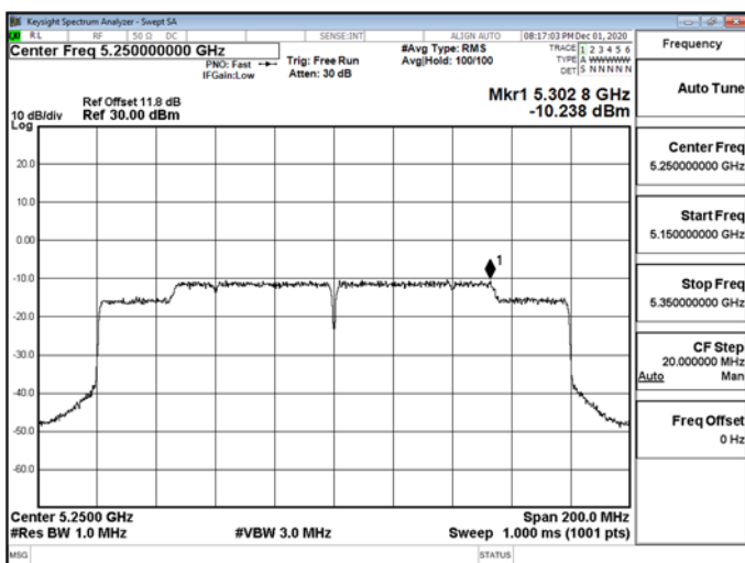
802.11ax_160MHz_5250MHz-5250
