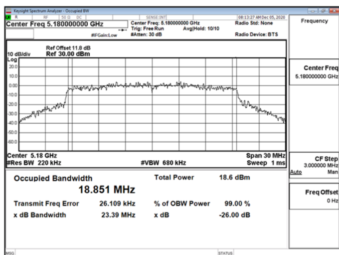
802.11ax_20MHz_Chain0_5180MHz
