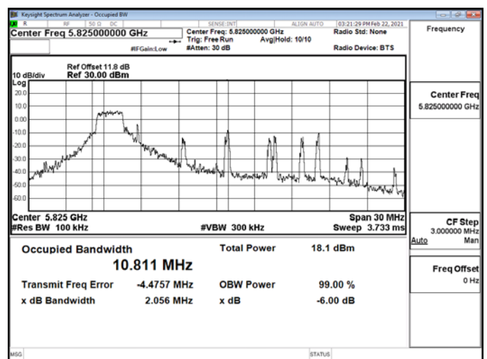
802.11ax_20MHz_Chain0_5825MHz_RU26_0
