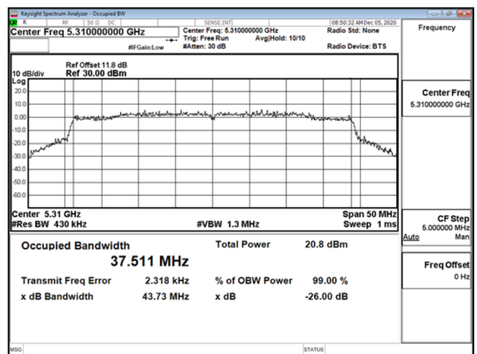
802.11ax_40MHz_Chain1_5310MHz
