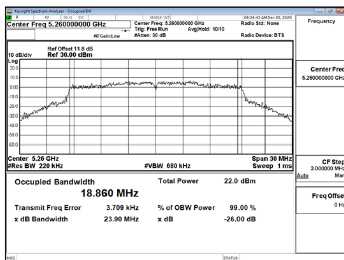
802.11ax_20MHz_Chain0_5260MHz
