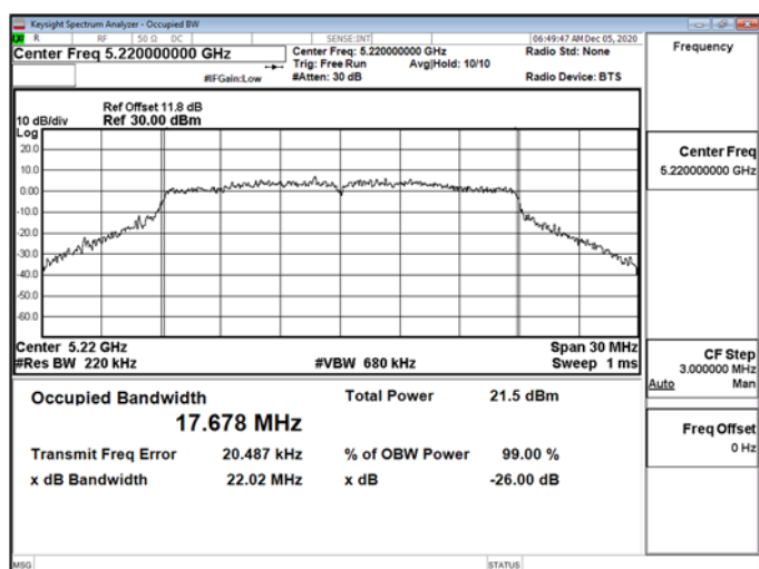
802.11n_20MHz_Chain1_5220MHz
