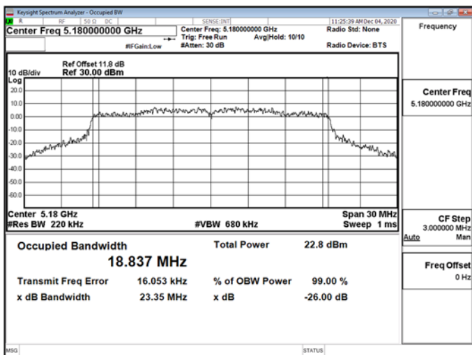
802.11ax_20MHz_Chain1_5180MHz
