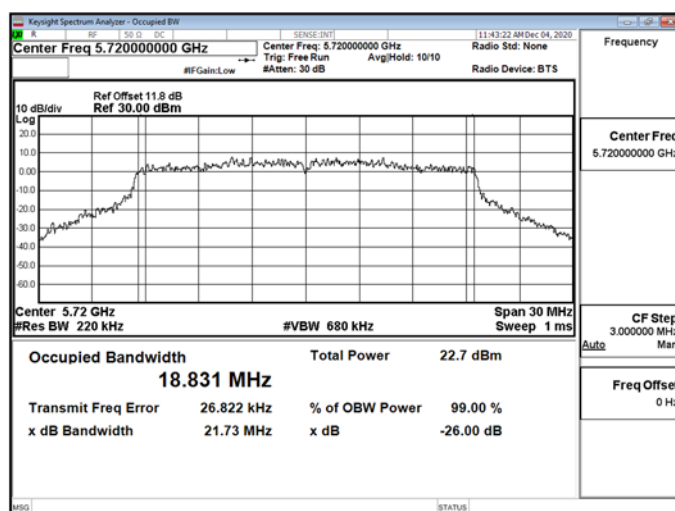
802.11ax_20MHz_Chain1_5720MHz
