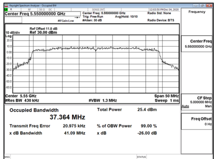
802.11ax_40MHz_Chain1_5550MHz
