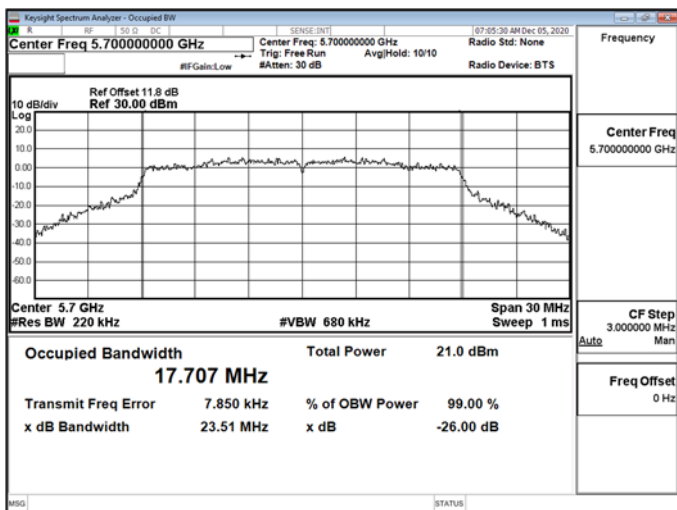
802.11n_20MHz_Chain0_5700MHz
