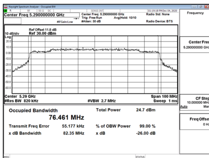
802.11ax_80MHz_Chain1_5290MHz
