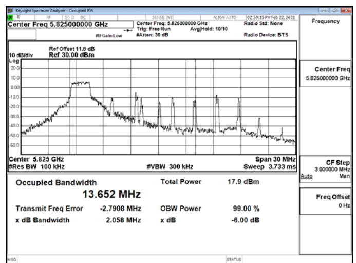
802.11ax_20MHz_Chain1_5825MHz_RU26_0
