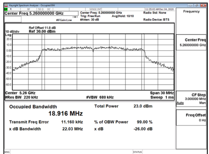
802.11ax_20MHz_Chain1_5260MHz
