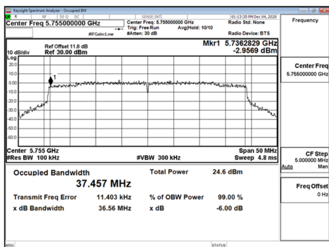
802.11ax_40MHz_Chain1_5755MHz
