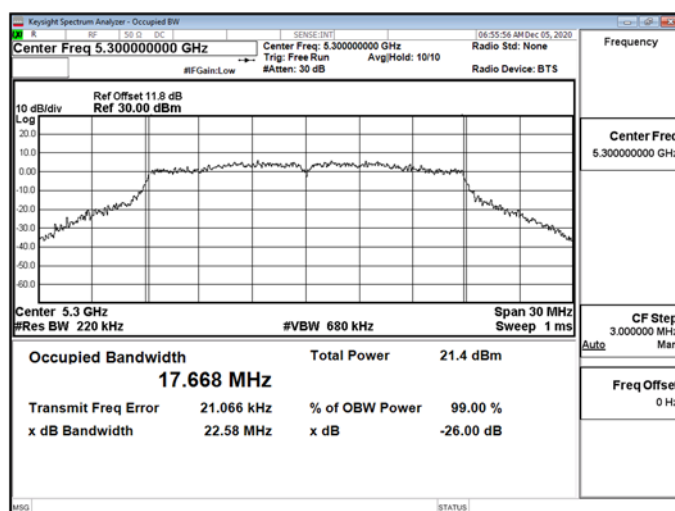
802.11n_20MHz_Chain1_5300MHz
