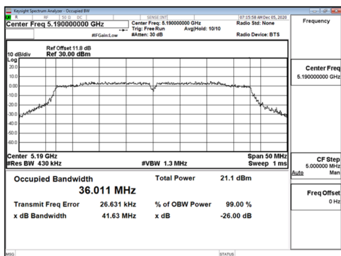
802.11n_40MHz_Chain0_5190MHz
