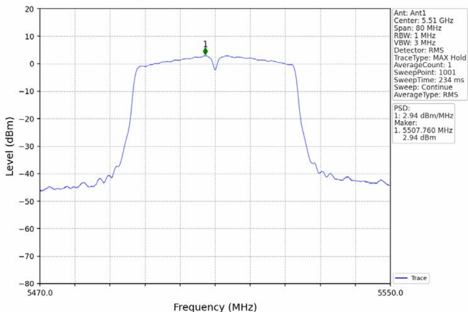
802.11n(HT40)_LCH_5510MHz_Ant1_NTNV
