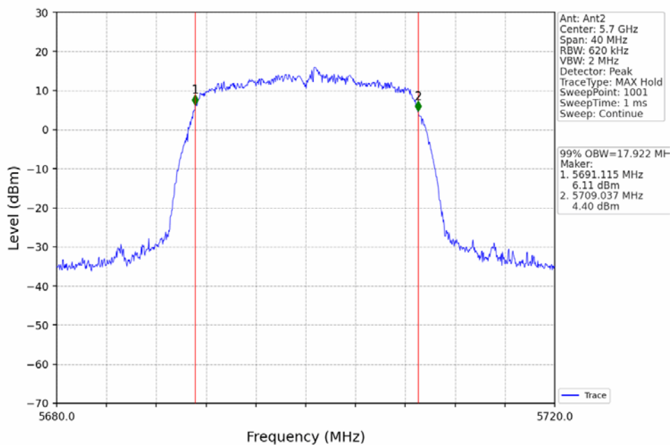
802.11n(HT20)_HCH_5700MHz_Ant2_NTNV
