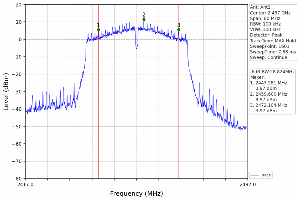
11N40_MCH_2457MHz_Ant2_NTNV
