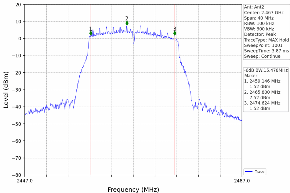
11G_MCH_2467MHz_Ant2_NTNV
