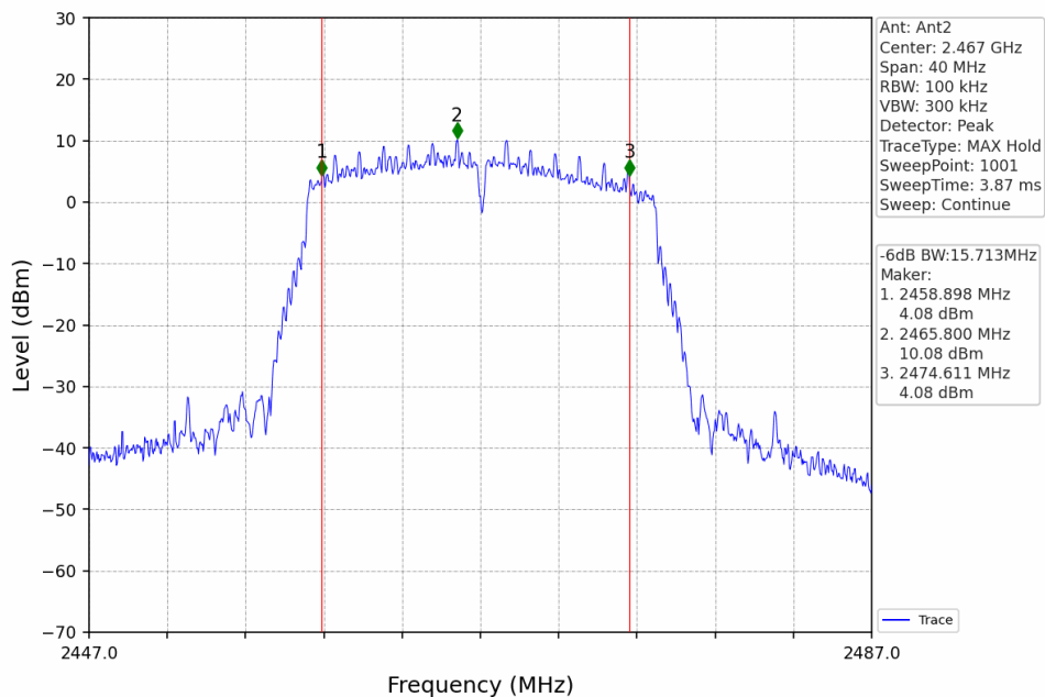
11N20_MCH_2467MHz_Ant2_NTNV
