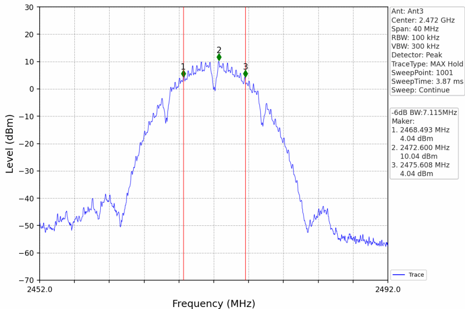
11B_HCH_2472MHz_Ant3_NTNV
