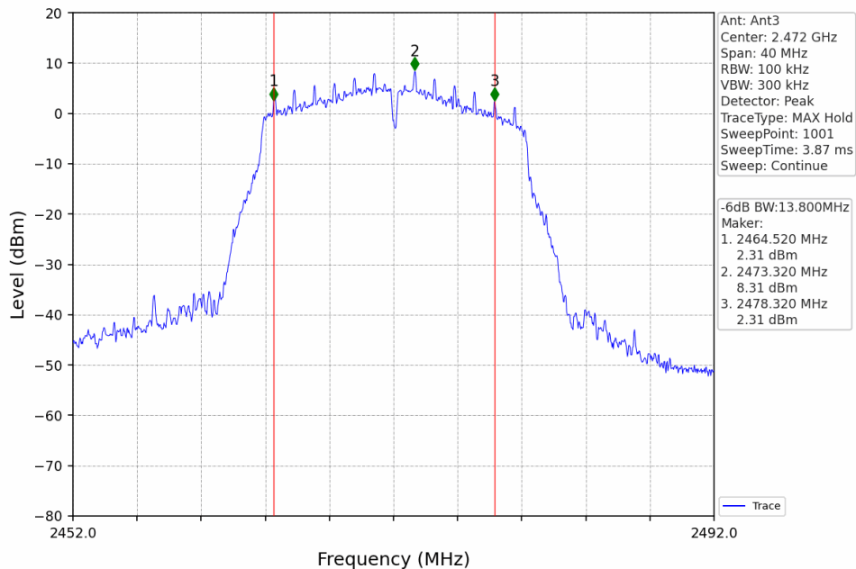
11G_HCH_2472MHz_Ant3_NTNV
