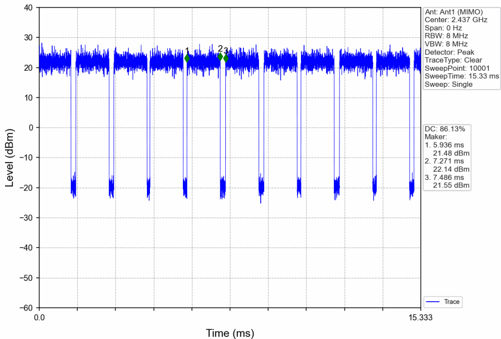
802.11n(HT20)_MCH_2437MHz_Ant1 (MIMO)_NTNV
