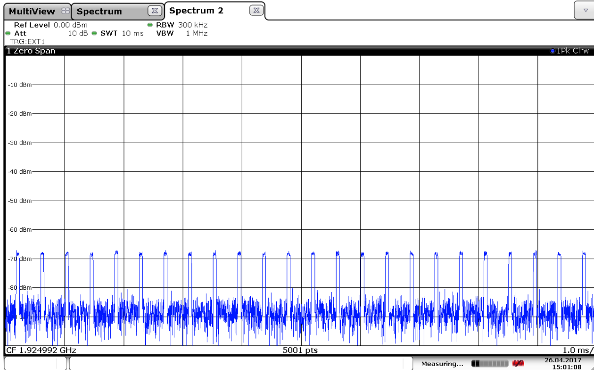
50 µs Pulses
