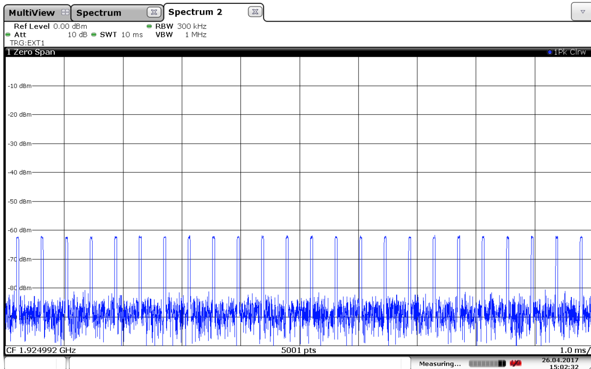
35 µs Pulses
