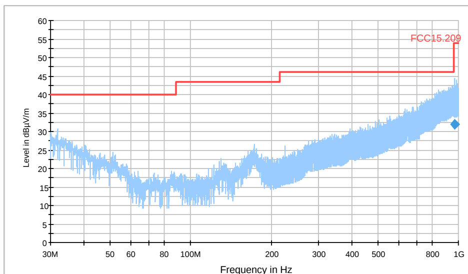
01_FCC15.209_hor+vert_kipp
