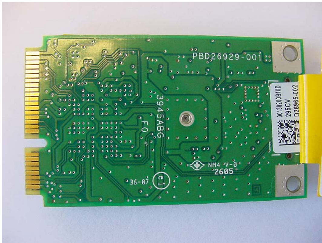
WLAN module (Rear)
