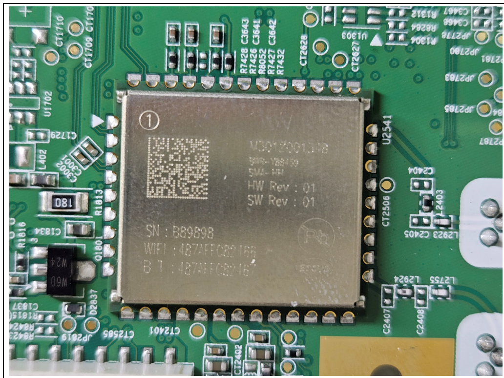
<WLAN Module>
