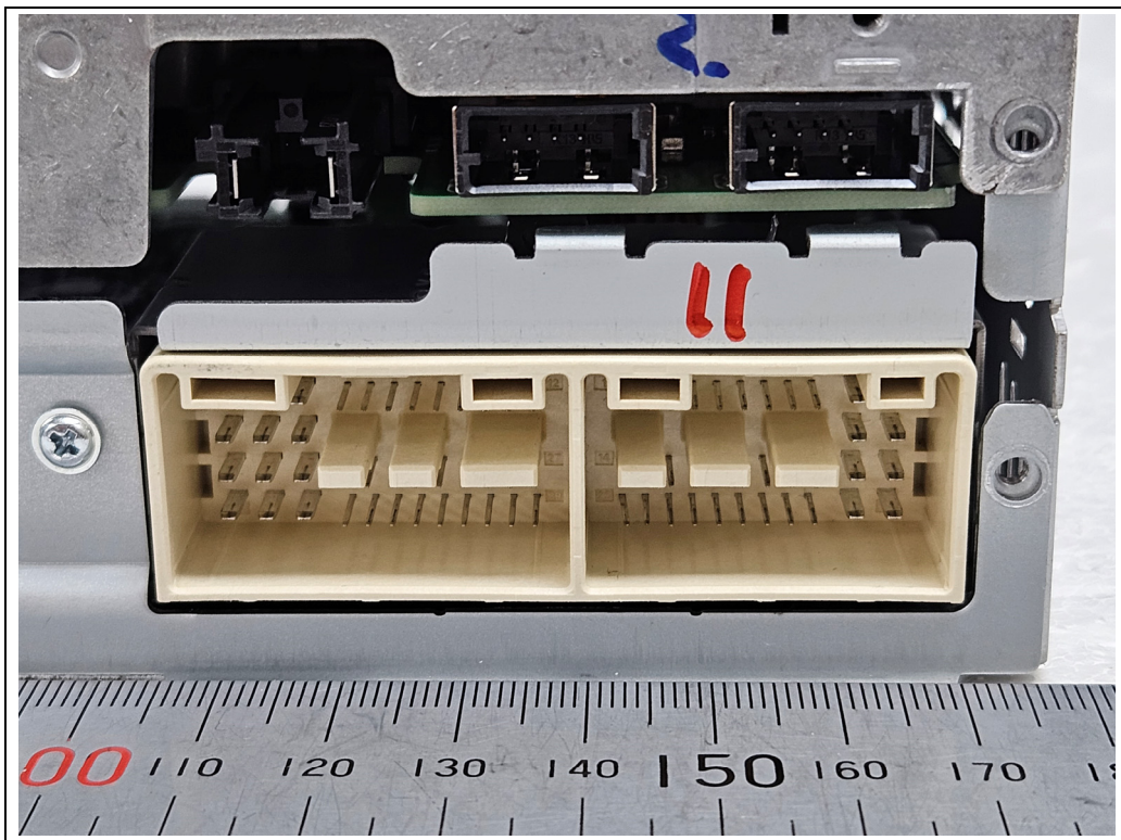
<Port 1>
