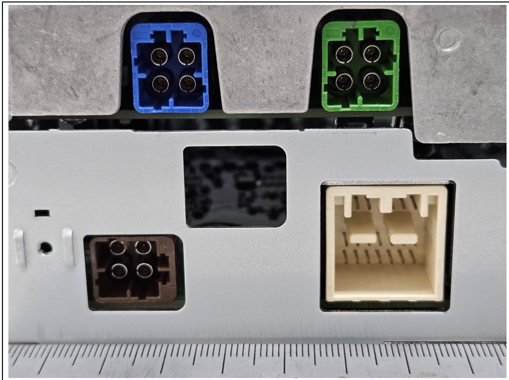
<Port 2>
