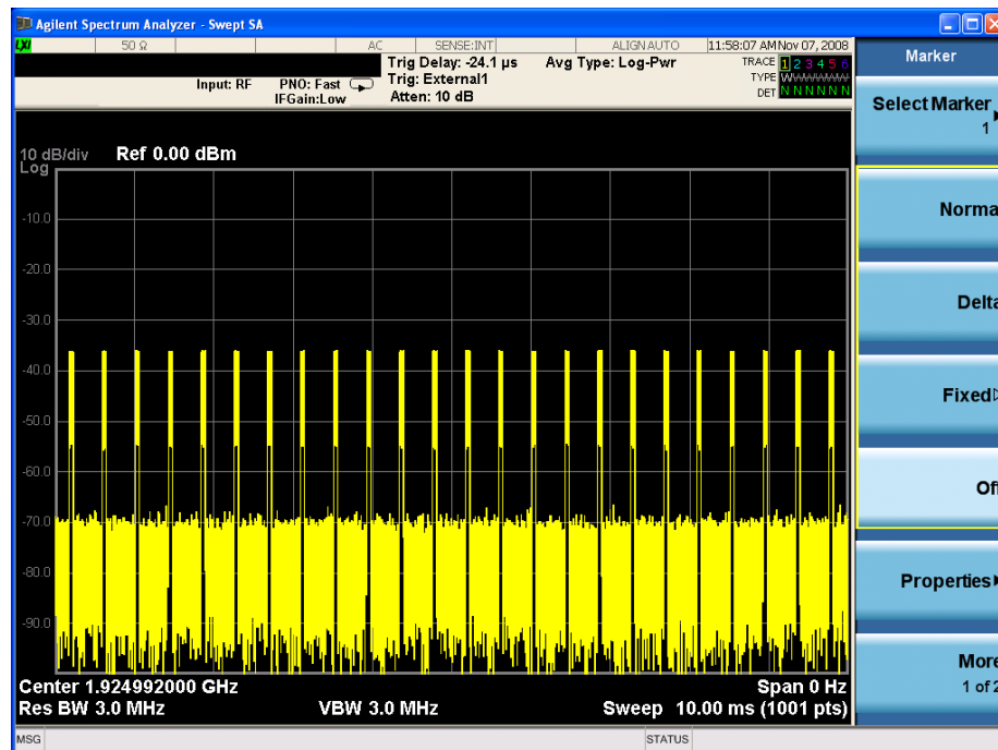
50 µs Pulses
