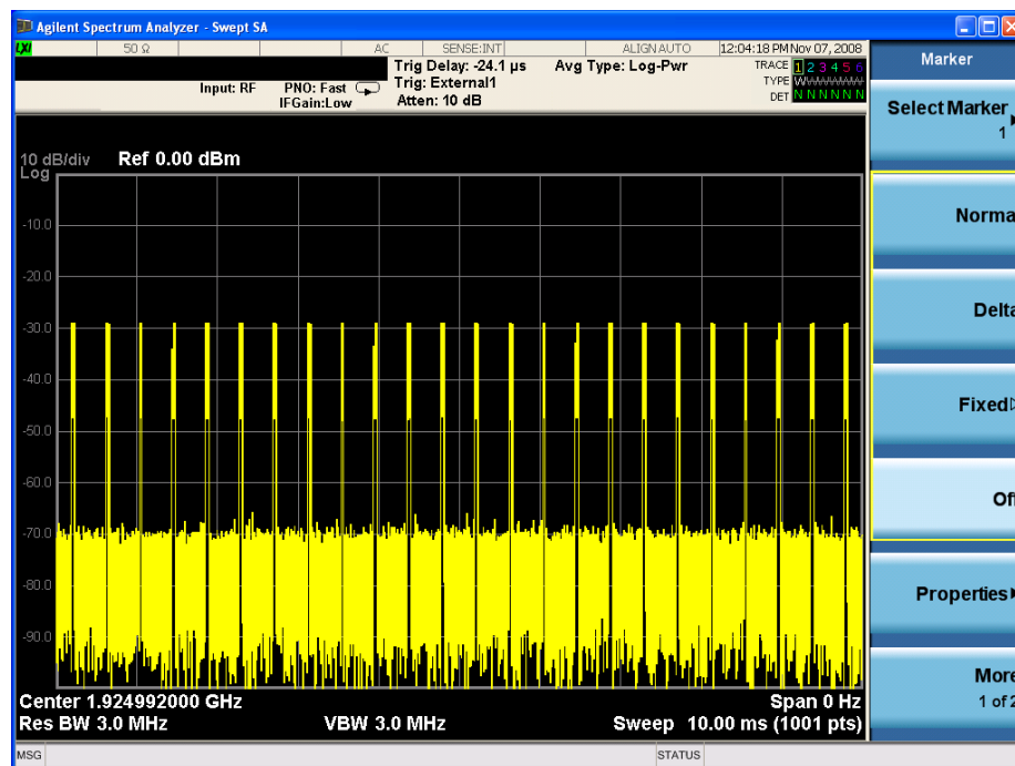
35 µs Pulses
