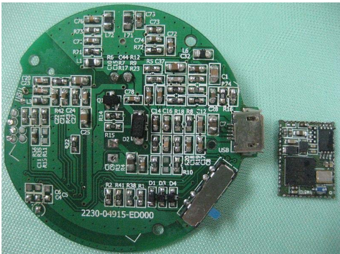
PCB-A
