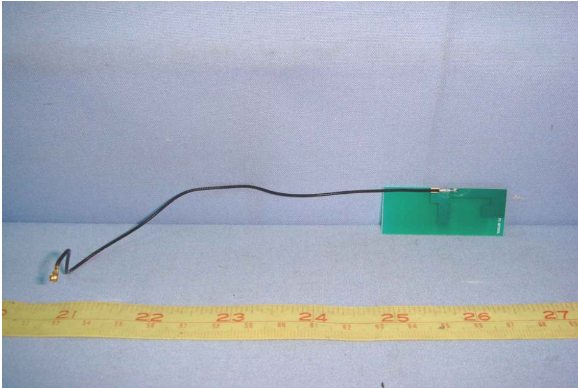
PIFA Antenna
