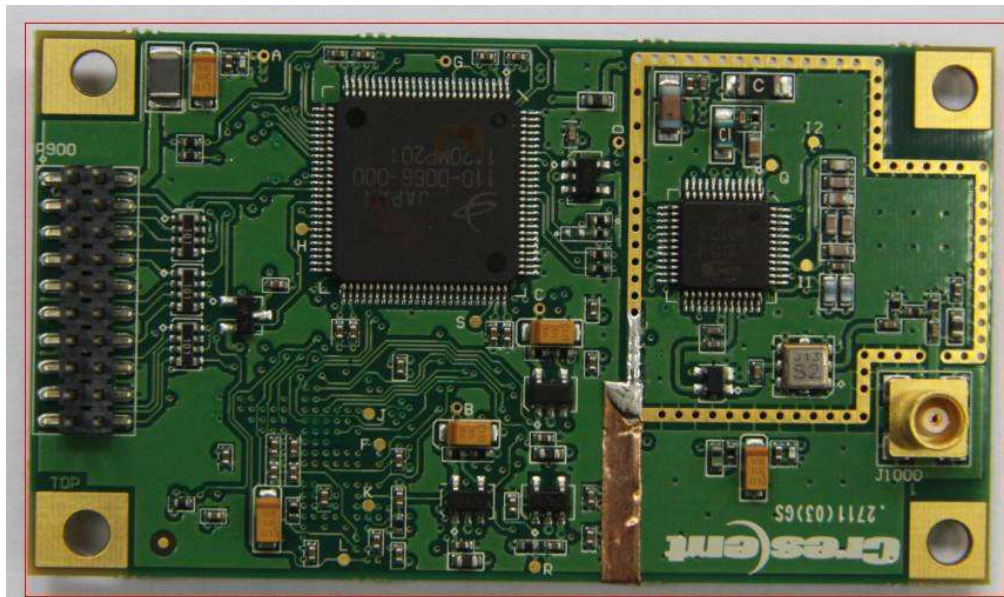
GPS Module Bottom
