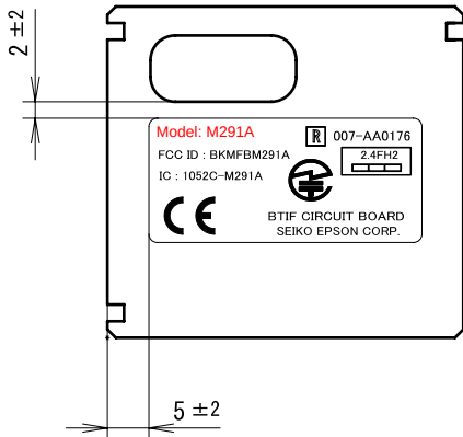
BT基板Label貼り付け位置 (貼り付け面（B面）から見た位置)
