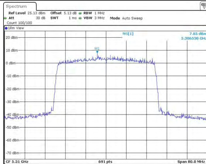
11AX40MIMO_Ant2_5310
