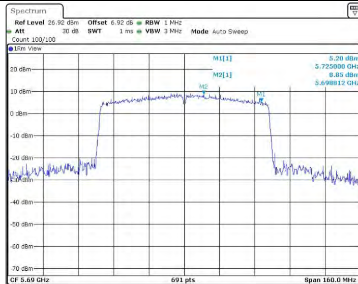
11AC80SISO_Ant1_5690_UNII-2C
