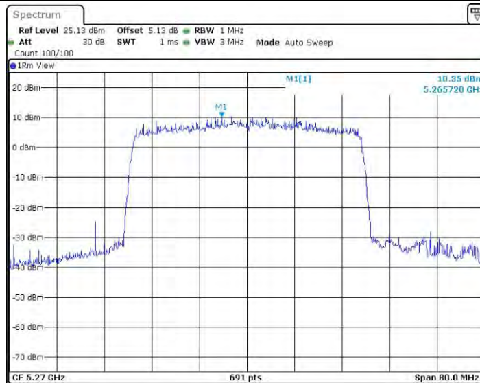
11AX40SISO_Ant2_5270
