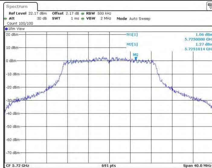
11N20MIMO_Ant1_5720_UNII-3
