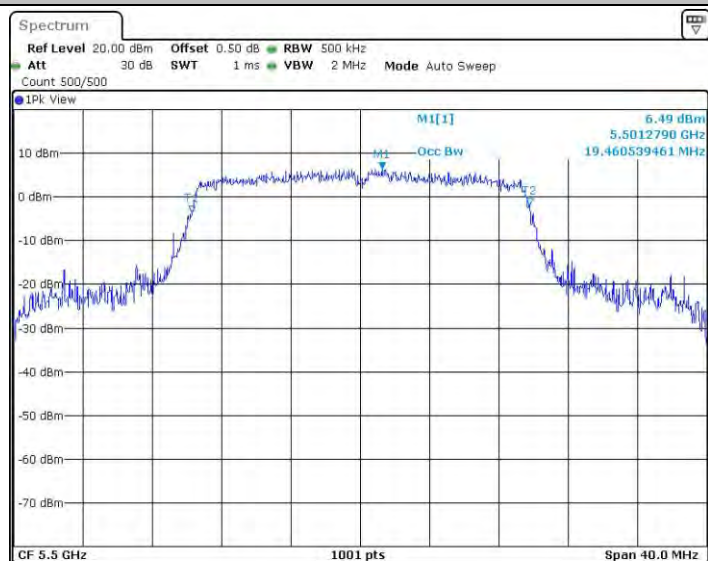
11AX20SISO_Ant1_5500
