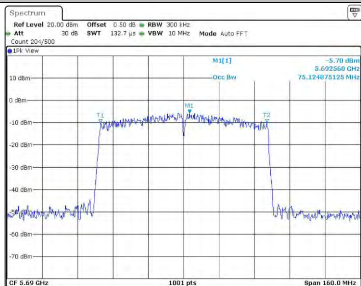
11AC80MIMO_Ant2_5690
