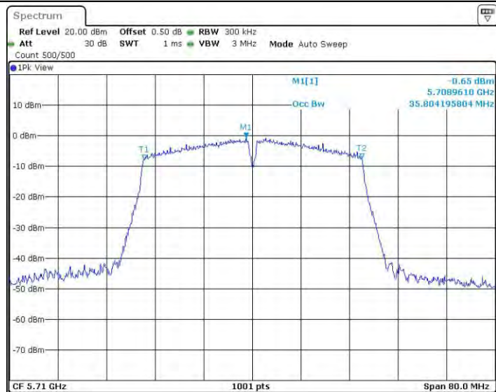
11AC40MIMO_Ant1_5710
