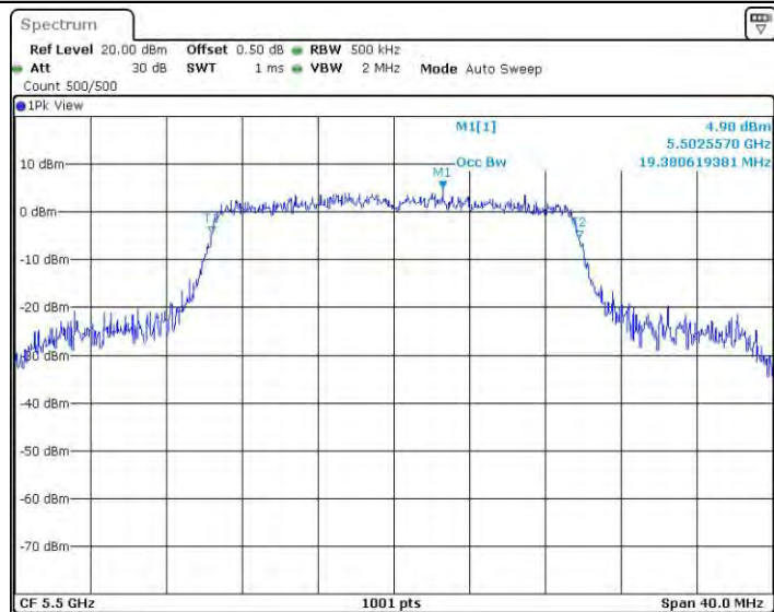
11AX20SISO_Ant2_5500
