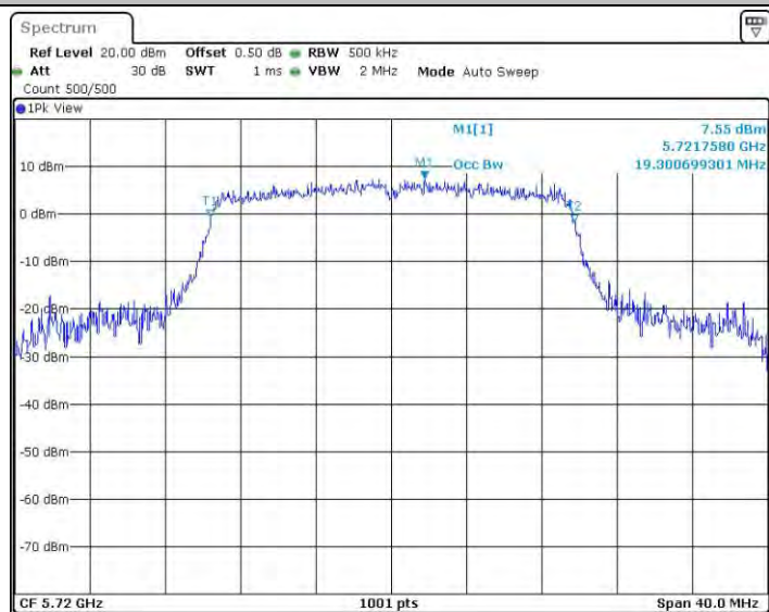
11AX20SISO_Ant2_5720
