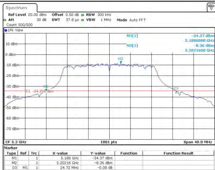
11N20MIMO_Ant1_5200
