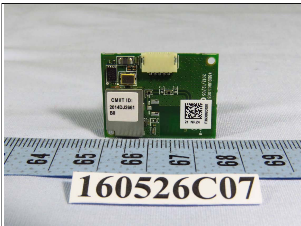
Module: DBUB-E207
