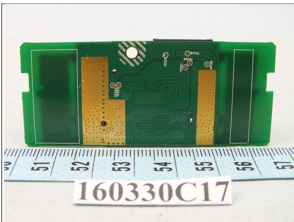
Module: WN7122BEP
