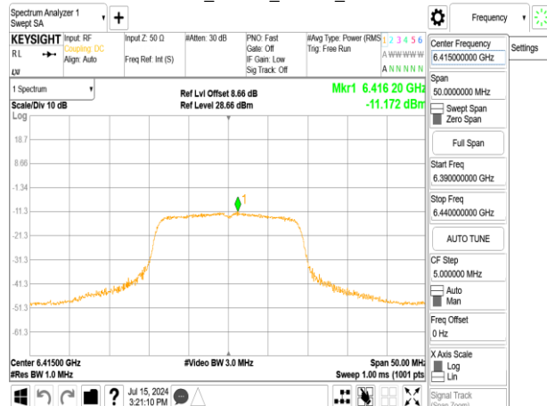
802.11n_20MHz_Chain1_6415MHz
