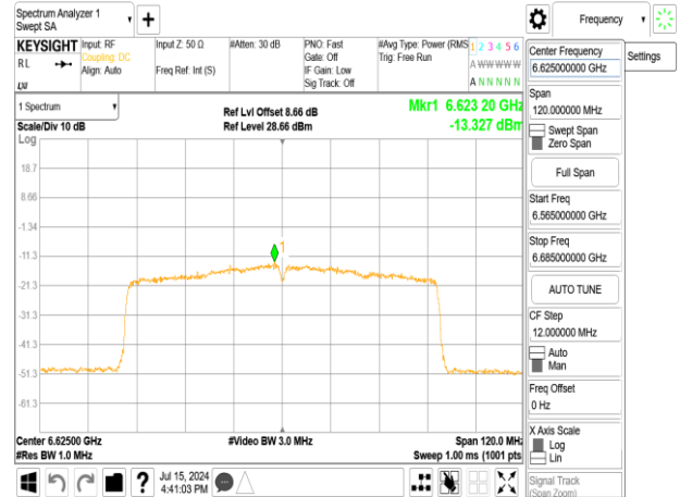
802.11ac_80MHz_Chain0_6625MHz
