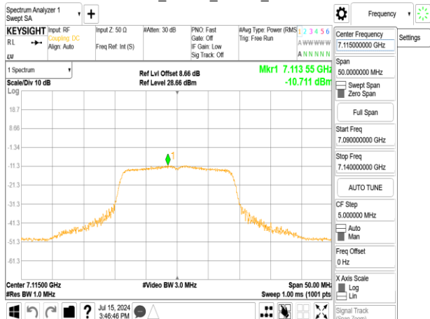
802.11n_20MHz_Chain0_7115MHz
