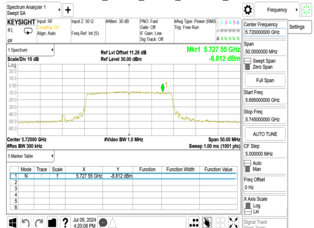
802.11ax_20MHz_Chain1_5720MHz_UNII 3
