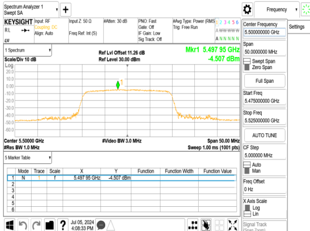
802.11ax_20MHz_Chain1_5500MHz_RU106_53
