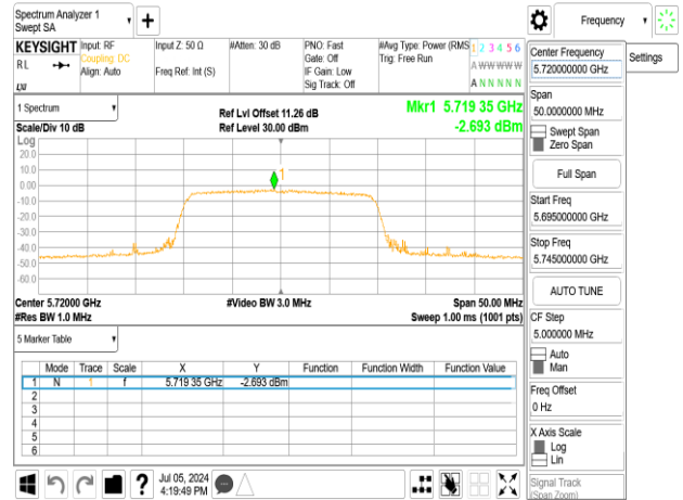
802.11ax_20MHz_Chain1_5720MHz_UNII 3
