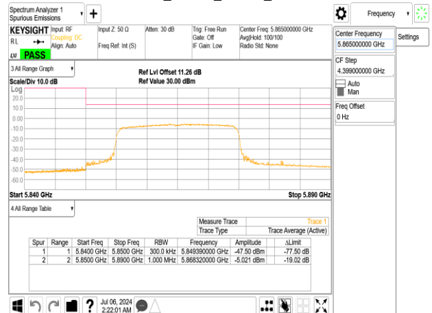
802.11ax_20MHz_Chain0_5865MHz
