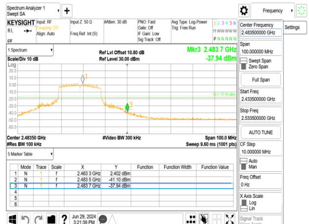
802.11ax_20MHz_Chain0_2462MHz
