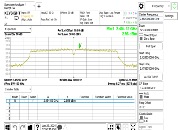
802.11n_40MHz_Chain1_2452MHz
