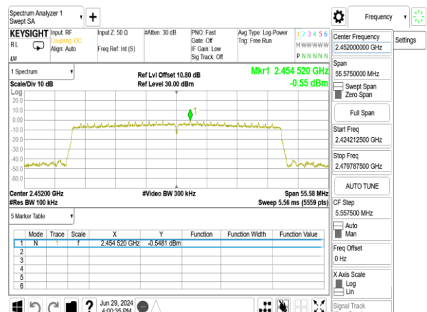
802.11ax_40MHz_Chain1_2452MHz
