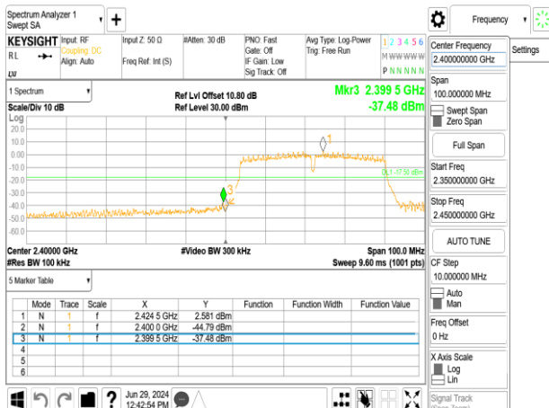
802.11n_40MHz_Chain1_2422MHz
