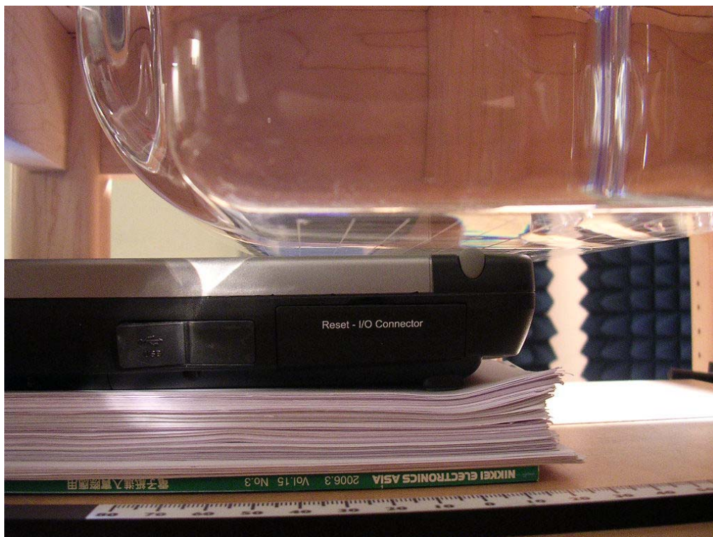
EUT Back
