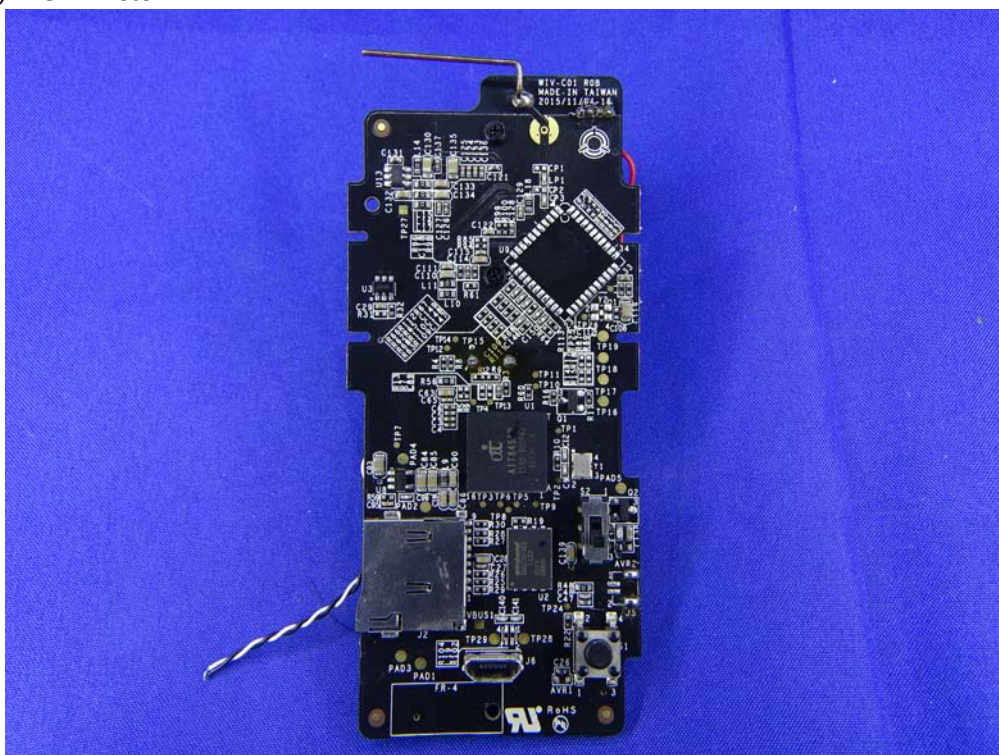
(14) EUT Photo
