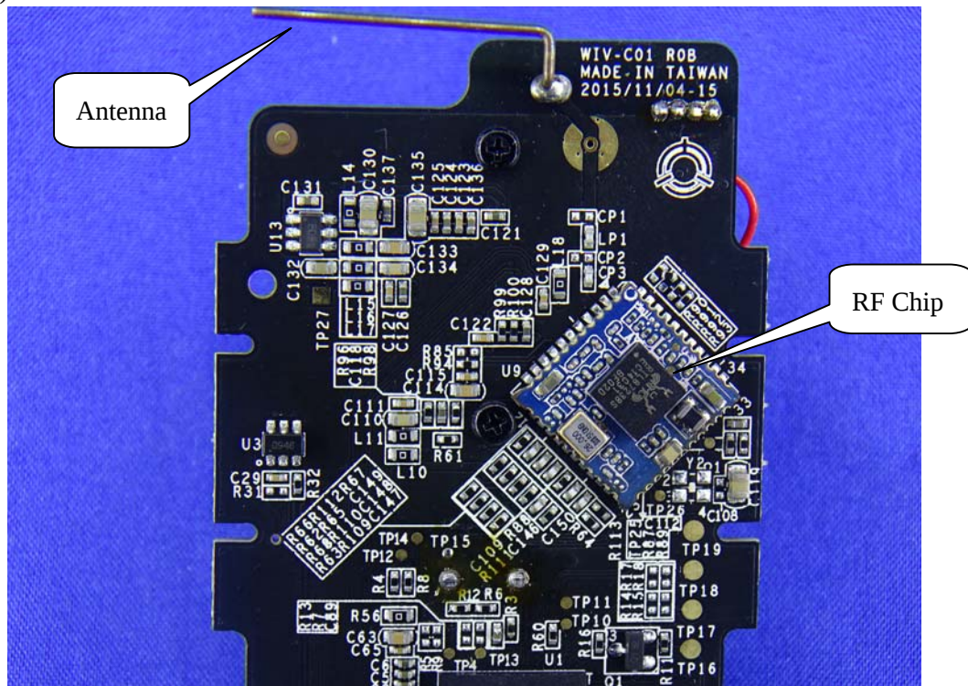
(17) EUT Photo
