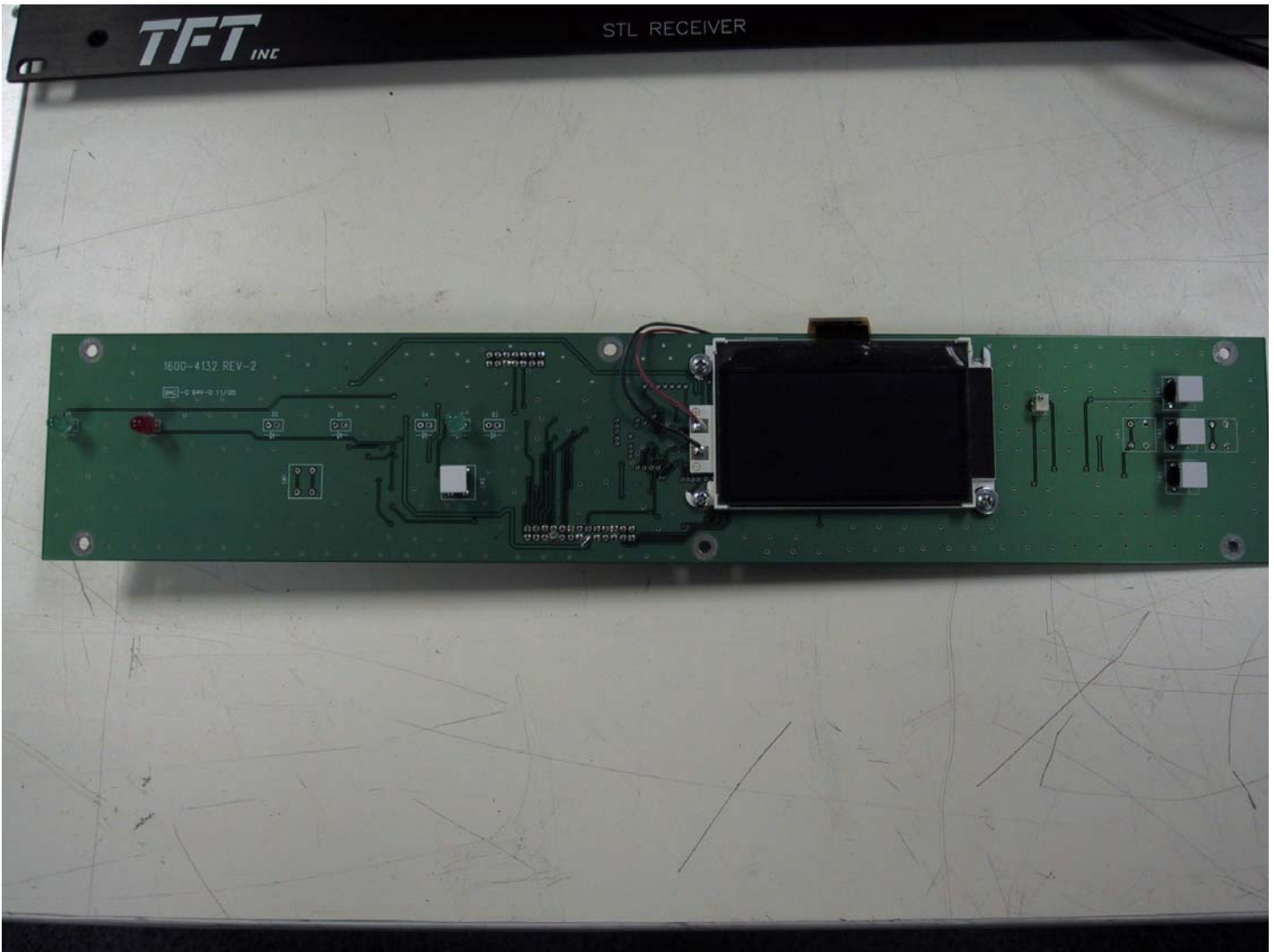
Display PCB – Bottom
