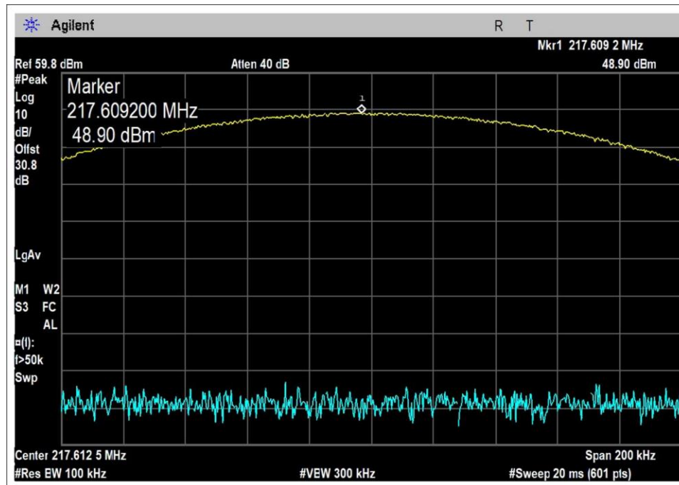
217.6125MHz, Pi/8-16
