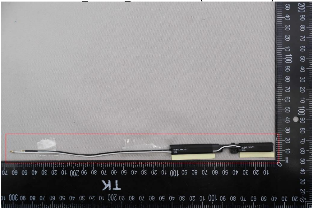
BT&amp;WIFI_Antenna_AYF6Y-200008 (1415-0ADV000)
