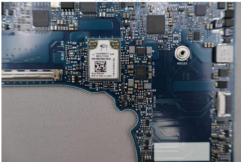
WLAN Module
