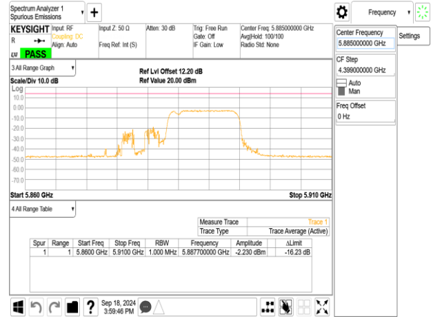
802.11be_20MHz_ChainB_5885MHz_52+26_MRU3
