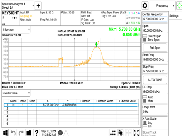
802.11be_20MHz_ChainB_5700MHz_RU26_8
