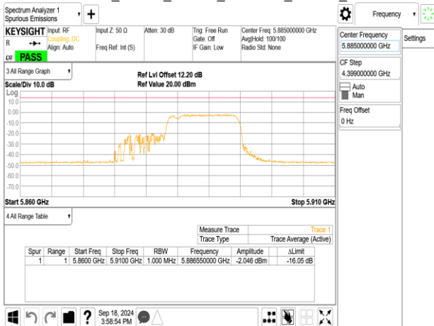
802.11be_20MHz_ChainA_5885MHz_52+26_MRUI3
