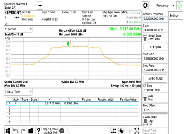
802.11be_20MHz_ChainB_5220MHz
