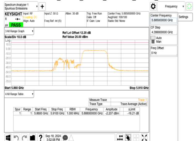
802.11be_20MHz_ChainB_5885MHz_RU106_54
