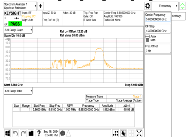
802.11be_20MHz_ChainA_5885MHz_RU52_40
