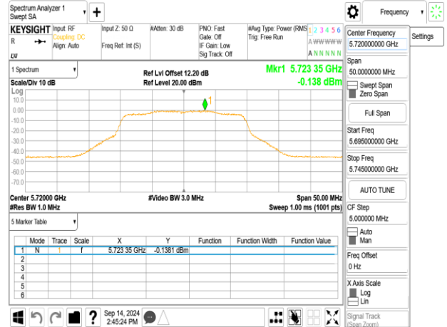
802.11be_20MHz_ChainB_5720MHz_UNII 3
