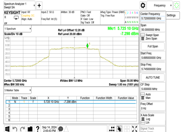
802.11be_20MHz_ChainB_5720MHz_UNII 3
