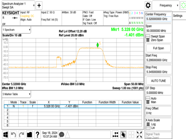
802.11be_20MHz_ChainB_5320MHz_RU26_8
