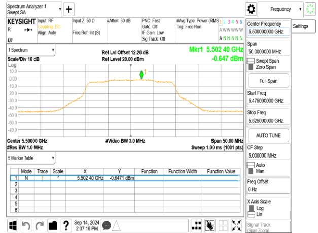
802.11be_20MHz_ChainB_5500MHz_106+26_MRU1
