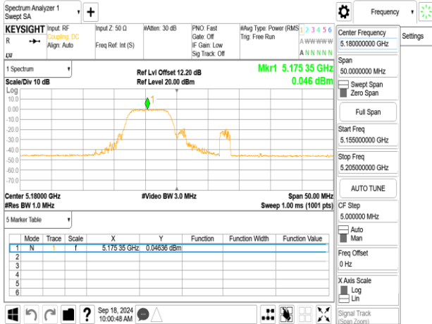
802.11be_20MHz_ChainB_5180MHz_RU106_53
