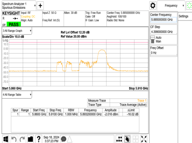
802.11be_20MHz_ChainB_5885MHz_RU52_40
