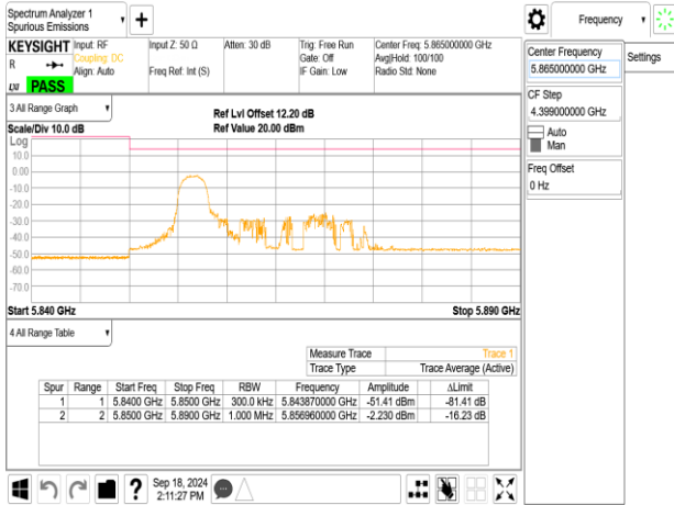
802.11be_20MHz_ChainB_5865MHz_RU52_37
