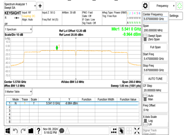
802.11ax_160MHz_ChainA_5570MHz_RU996_67
