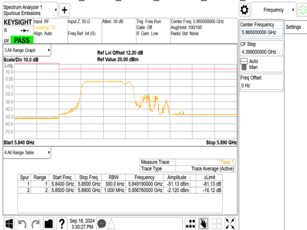
802.11be_20MHz_ChainA_5865MHz_52+26_MRUI1
