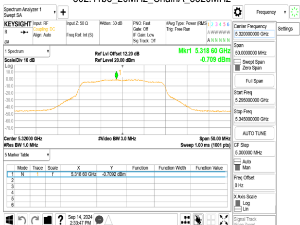
802.11be_20MHz_ChainA_5320MHz_106+26_MRU2
