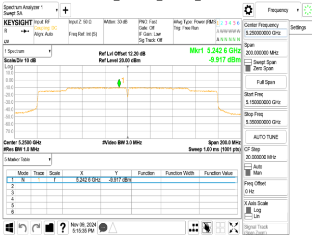
802.11ax_160MHz_ChainA_5250MHz_RU996_67
