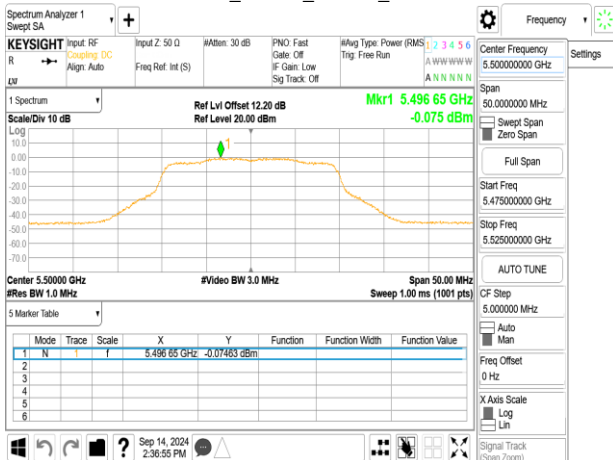
802.11be_20MHz_ChainA_5500MHz_106+26_MRU1
