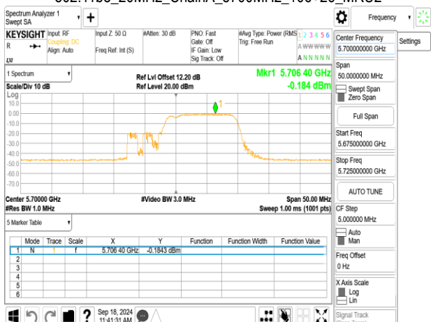
802.11be_20MHz_ChainA_5700MHz_106+26_MRUI2
