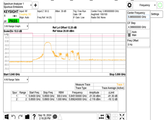
802.11be_20MHz_ChainA_5865MHz_RU52_37
