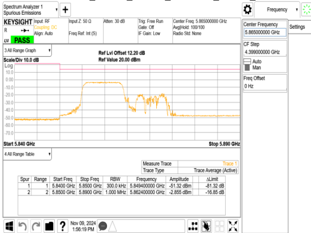
802.11ax_20MHz_ChainB_5865MHz_RU26_0
