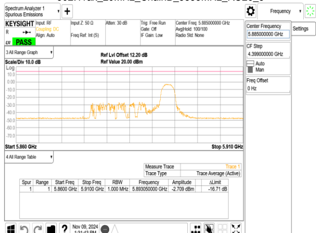
802.11ax_20MHz_ChainB_5885MHz_RU52_40
