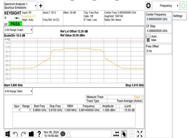
802.11ax_20MHz_ChainB_5885MHz_RU106_54
