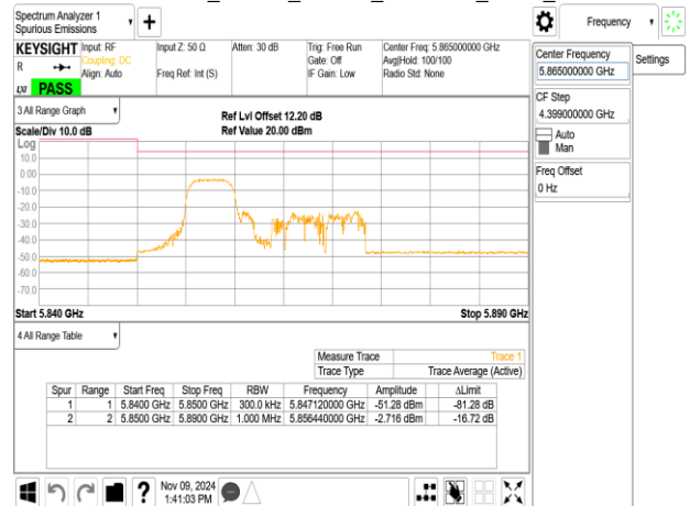
802.11ax_20MHz_ChainB_5885MHz
