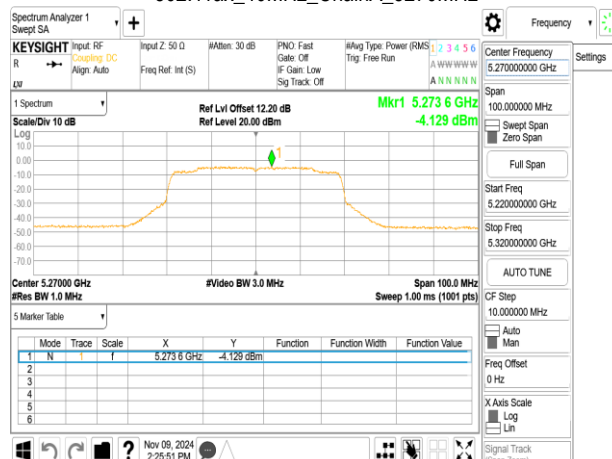
802.11ax_40MHz_ChainA_5270MHz
