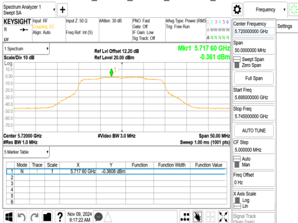
802.11ax_20MHz_ChainB_5720MHz_UNII 3
