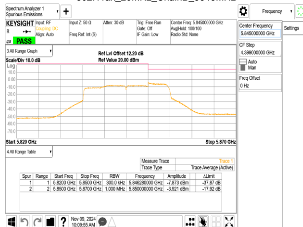
802.11ax_20MHz_ChainB_5845MHz
