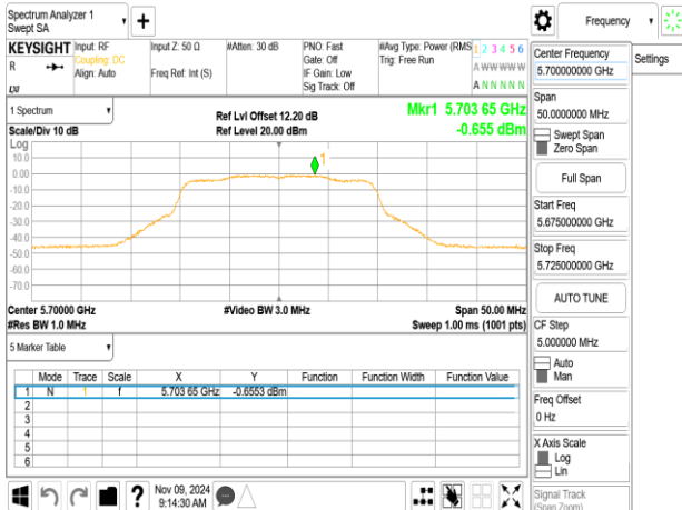
802.11ax_20MHz_ChainB_5700MHz
