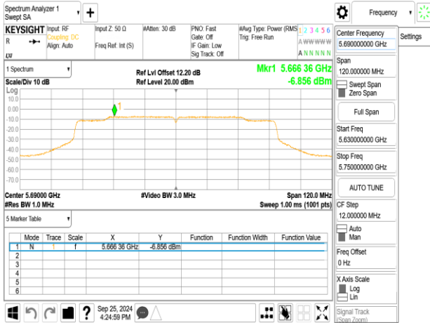
802.11ac_80MHz_ChainB_5690MHz_UNII 3
