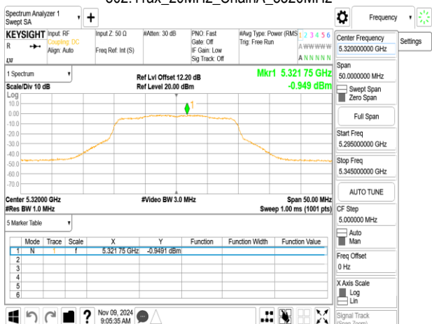
802.11ax_20MHz_ChainA_5320MHz_RU106_54
