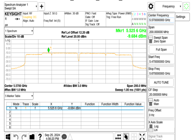
802.11ac_160MHz_ChainA_5570MHz
