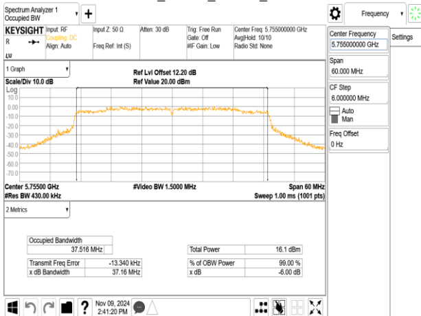
802.11ax_40MHz_ChainA_5755MHz_RU242_61
