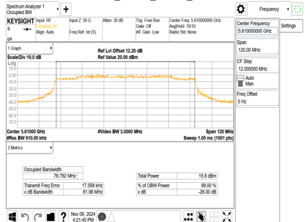
802.11ax_80MHz_ChainB_5610MHz
