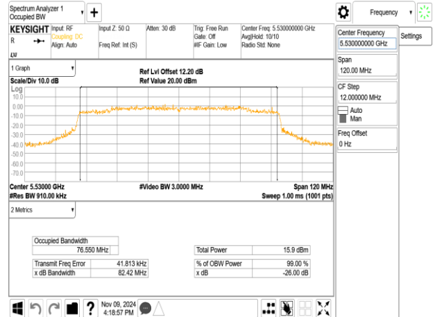
802.11ax_80MHz_ChainB_5530MHz_RU484_65
