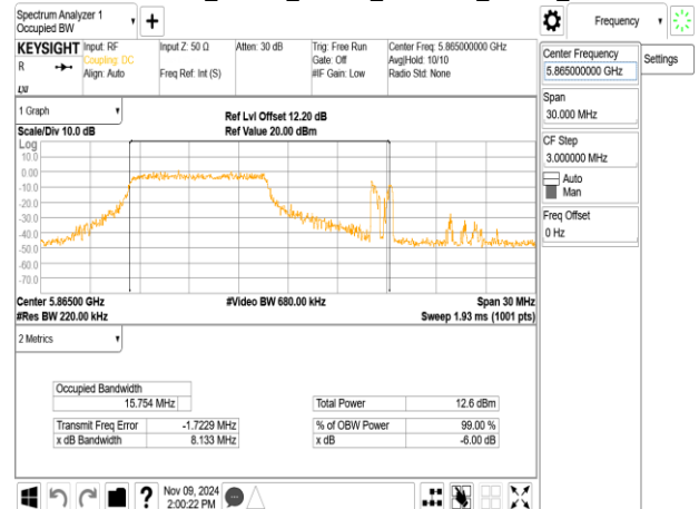
802.11ax_20MHz_ChainB_5865MHz_RU106_53
