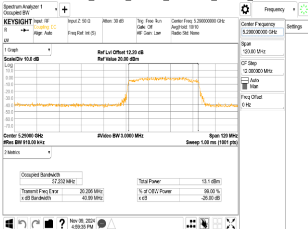
802.11ax_80MHz_ChainB_5290MHz_RU484_66
