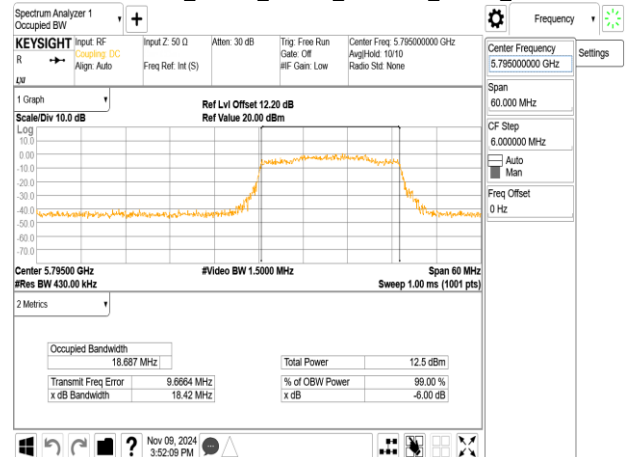
802.11ax_40MHz_ChainB_5795MHz_RU242_62
