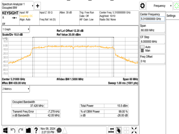
802.11ax_40MHz_ChainB_5310MHz_RU242_62
