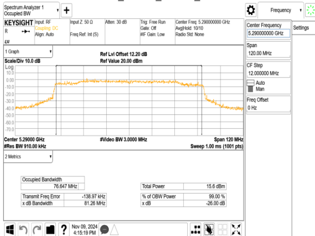
802.11ax_80MHz_ChainA_5290MHz_RU484_66
