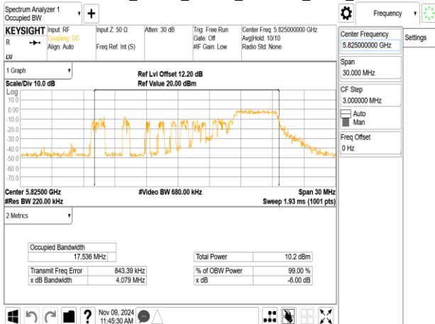
802.11ax_20MHz_ChainB_5825MHz_RU52_40
