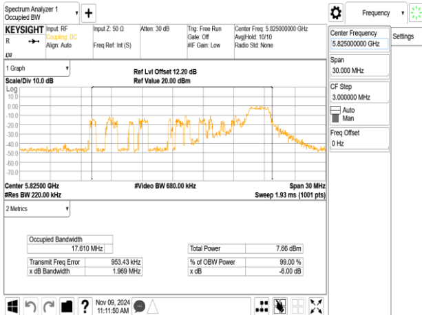
802.11ax_20MHz_ChainB_5825MHz_RU52_40
