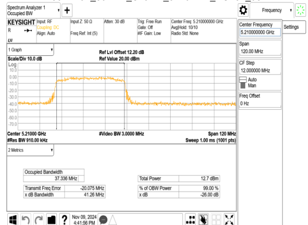
802.11ax_80MHz_ChainA_5210MHz_RU484_65
