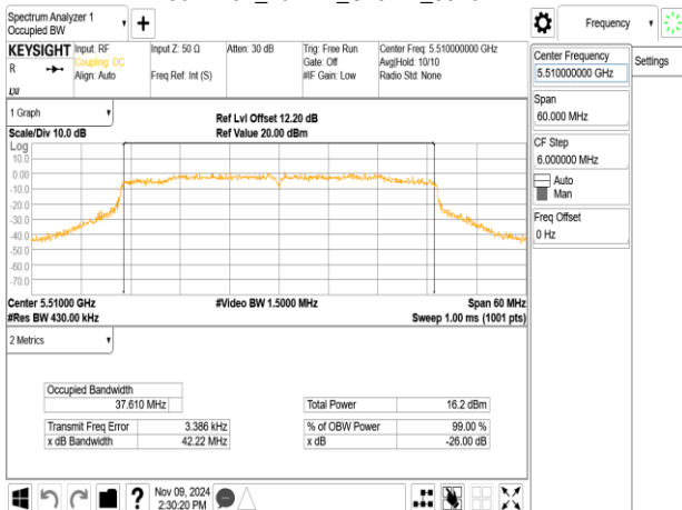
802.11ax_40MHz_ChainB_5510MHz
