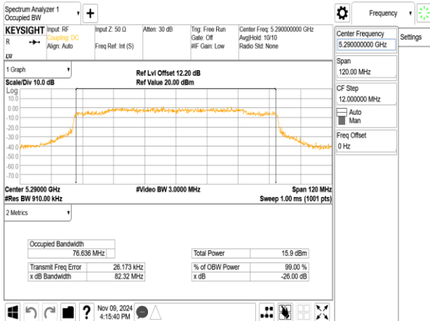
802.11ax_80MHz_ChainB_5290MHz_RU484_66
