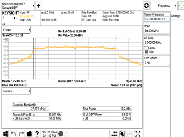
802.11ax_40MHz_ChainB_5755MHz
