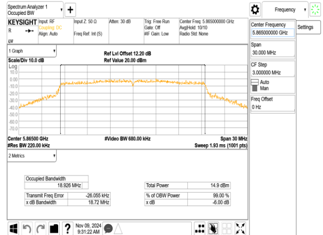
802.11ax_20MHz_ChainB_5865MHz_RU106_53
