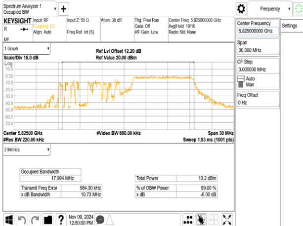
802.11ax_20MHz_ChainB_5825MHz_RU26_8
