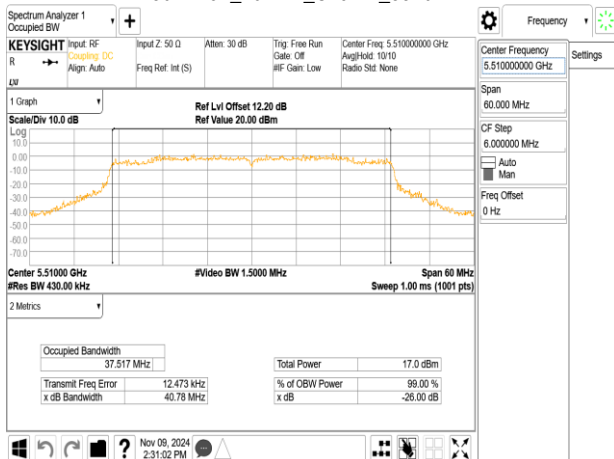
802.11ax_40MHz_ChainB_5510MHz
