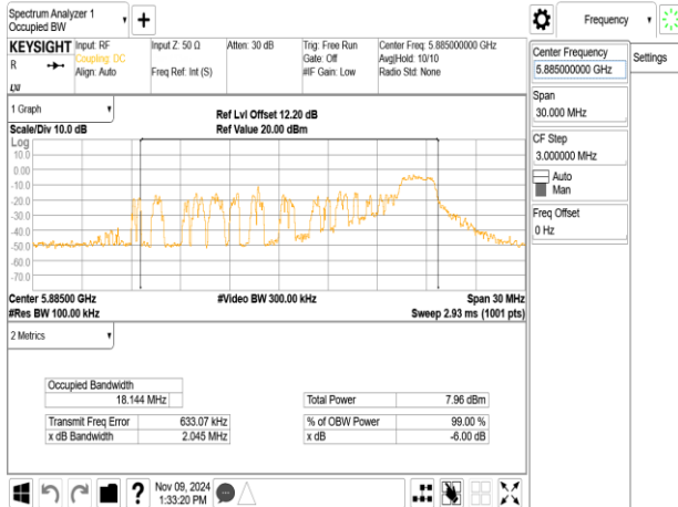
802.11ax_20MHz_ChainA_5885MHz_RU52_40
