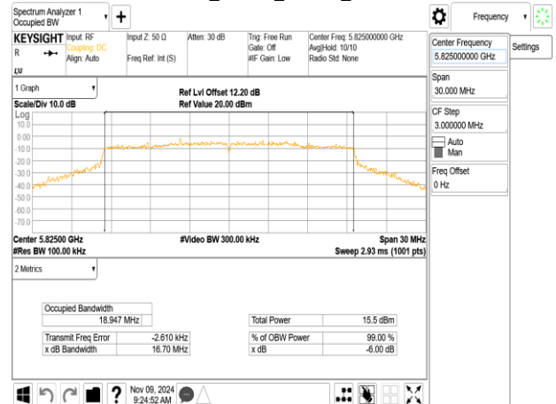
802.11ax_20MHz_ChainB_5825MHz
