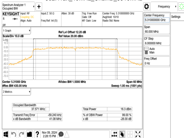
802.11ax_40MHz_ChainB_5310MHz_RU242_62
