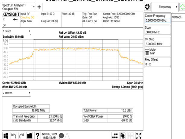
802.11ax_20MHz_ChainB_5260MHz
