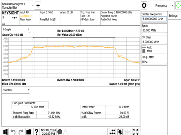
802.11ax_40MHz_ChainB_5190MHz
