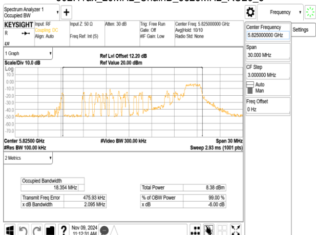
802.11ax_20MHz_ChainB_5825MHz_RU52_40
