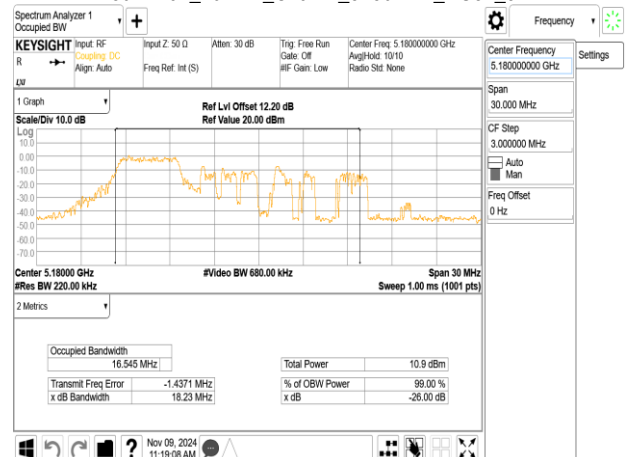
802.11ax_20MHz_ChainB_5180MHz_RU52_37
