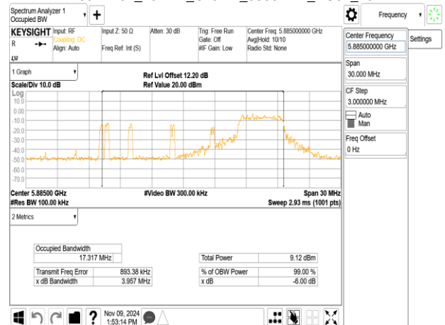
802.11ax_20MHz_ChainB_5885MHz_RU52_40
