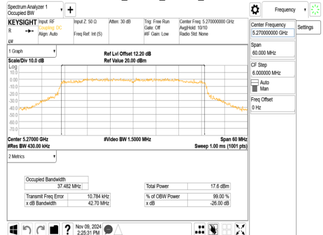
802.11ax_40MHz_ChainB_5270MHz
