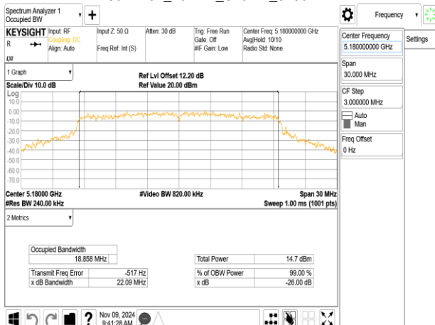
802.11ax_20MHz_ChainB_5180MHz
