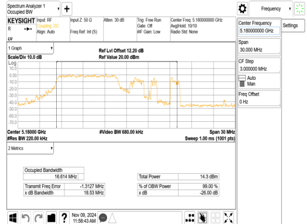
802.11ax_20MHz_ChainB_5180MHz_RU26_0
