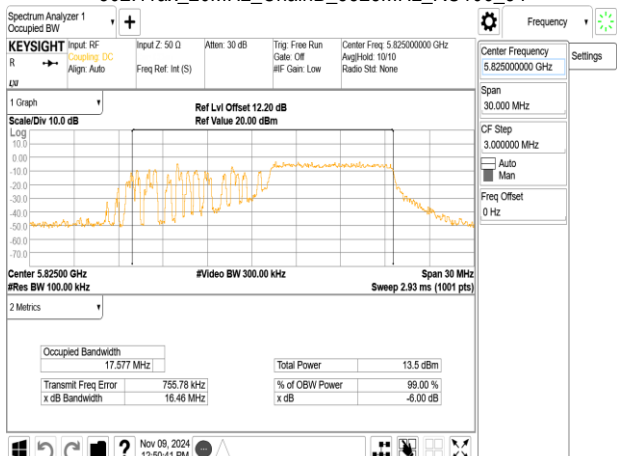
802.11ax_20MHz_ChainB_5825MHz_RU26_8
