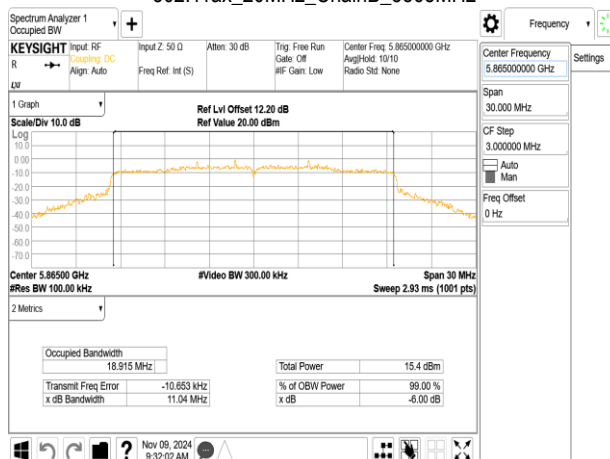
802.11ax_20MHz_ChainB_5865MHz_RU106_53
