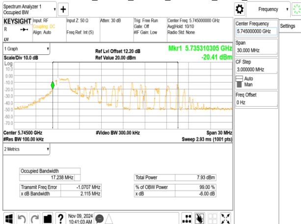
802.11ax_20MHz_ChainB_5745MHz_RU26_0
