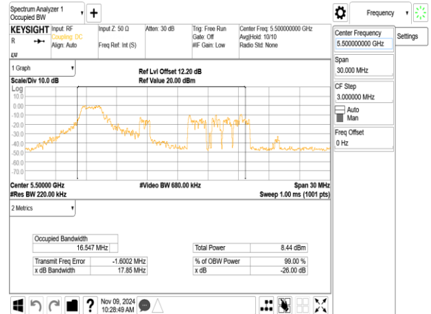
802.11ax_20MHz_ChainB_5500MHz_RU52_37
