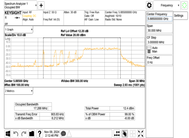
802.11ax_20MHz_ChainB_5885MHz_RU26_8
