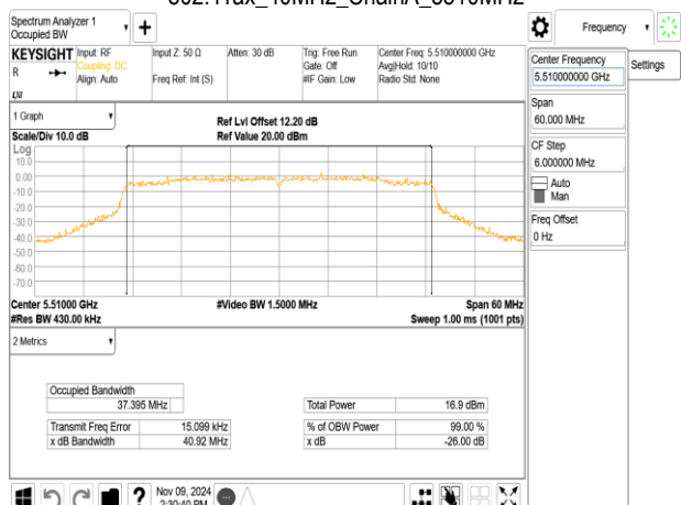
802.11ax_40MHz_ChainA_5510MHz_RU242_61
