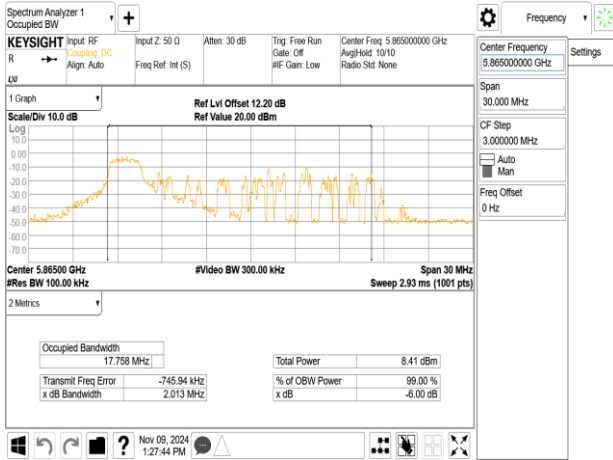
802.11ax_20MHz_ChainB_5865MHz_RU52_37
