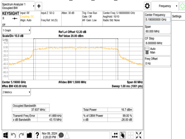
802.11ax_40MHz_ChainA_5190MHz_RU242_61
