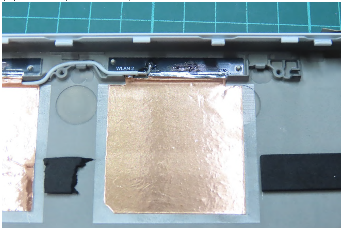
(30) EUT Photo (Antenna: INPAQ)
