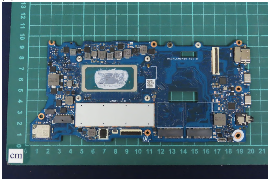
(16) EUT Photo
