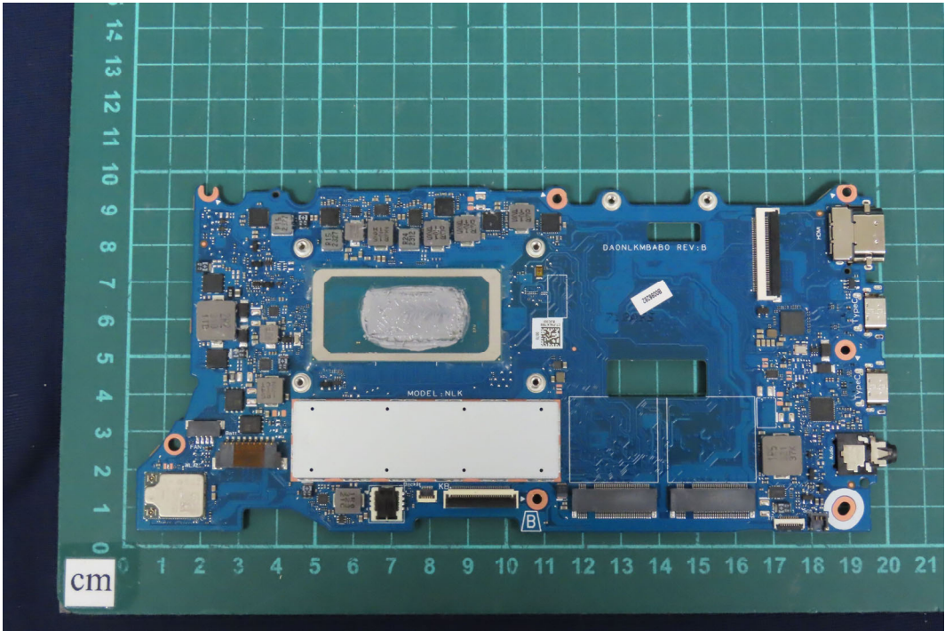
(17) EUT Photo
