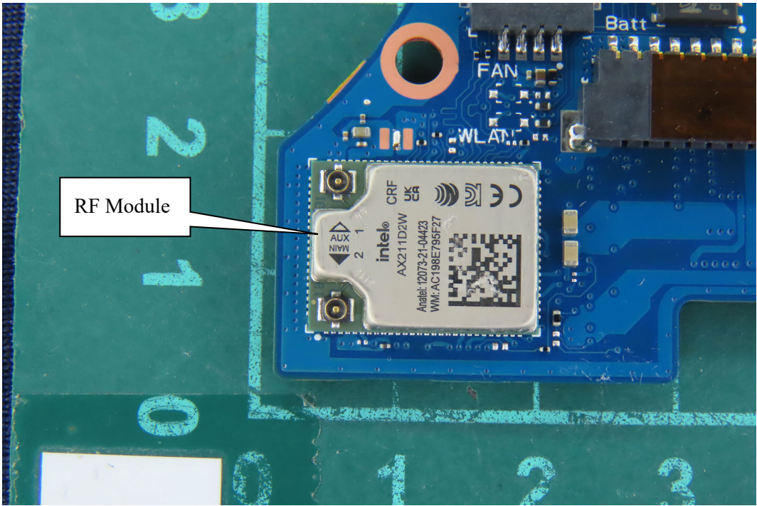
(18) EUT Photo
