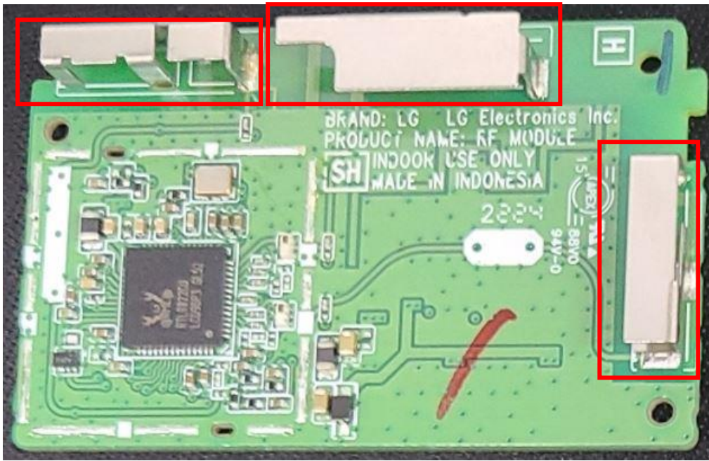
WLAN Ant1
