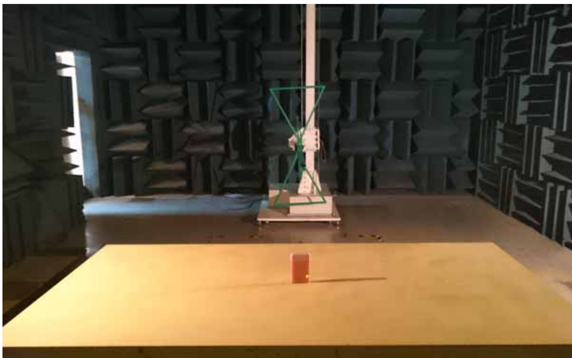
EUT on Stand
