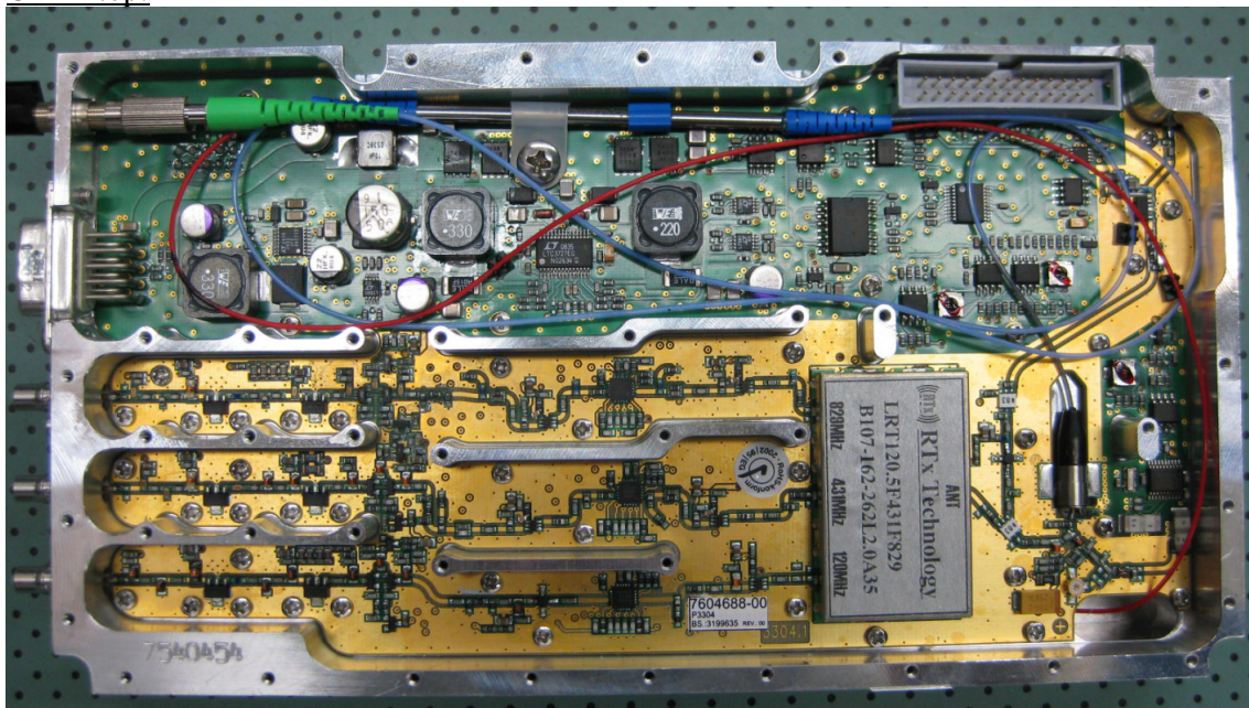
OTRx top:
