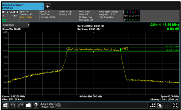
Figure 117 - 802.11ax HE20 SU Maximum 6 dB EBW
