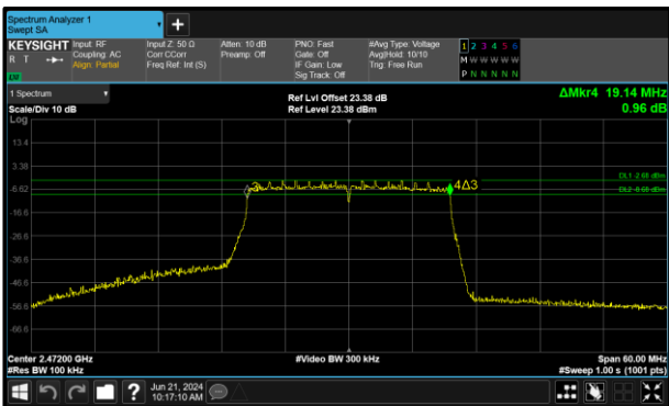
Figure 129 - 802.11ax HE20 SU Maximum 6 dB EBW
