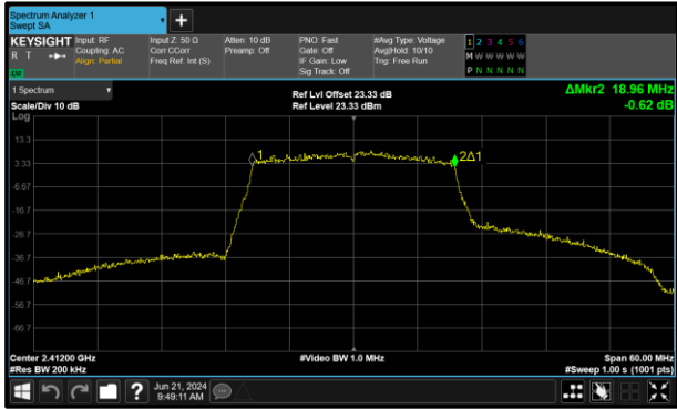
Figure 124 - 802.11ax HE20 SU Minimum 99% OBW
