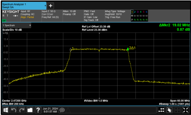
Figure 125 - 802.11ax HE20 SU Maximum 99% OBW
