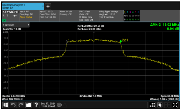
Figure 94 - 802.11ax HE20 SU Maximum 99% OBW
