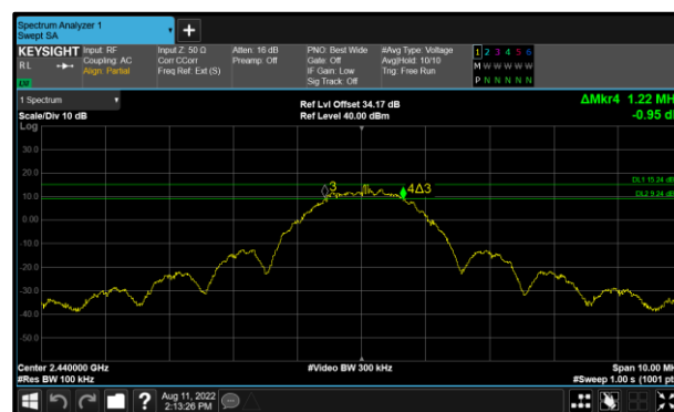
Figure 6 - Thread (D) 2440 MHz (CH18) 6 dB Bandwidth
