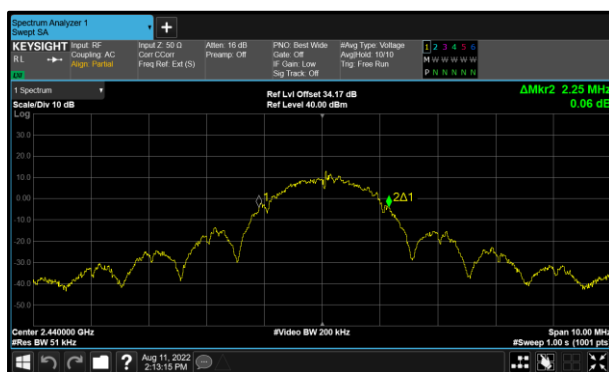
Figure 5 - Thread (D) 2440 MHz (CH18) 99% Bandwidth
