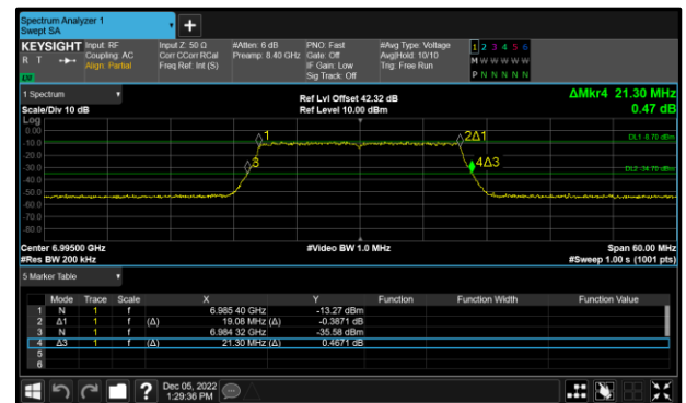
Figure 20 - 802.11ax HE20 SU Maximum 99% OBW
