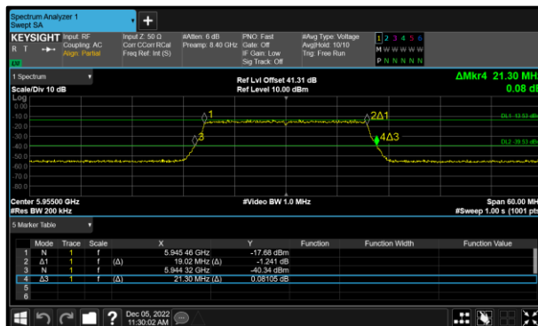
Figure 11 - 802.11ax HE20 SU Minimum 99% OBW
