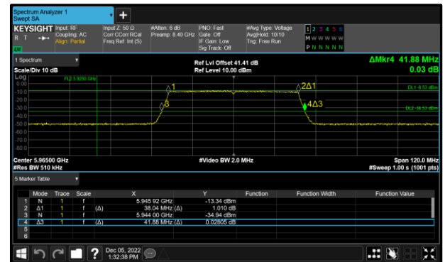
Figure 22 - 802.11ax HE40 SU Maximum 99% OBW
